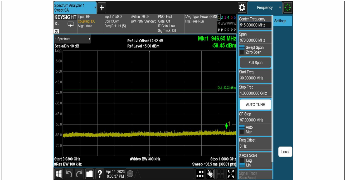
ZIGB-Ant1-2405-30~1000--2.23
