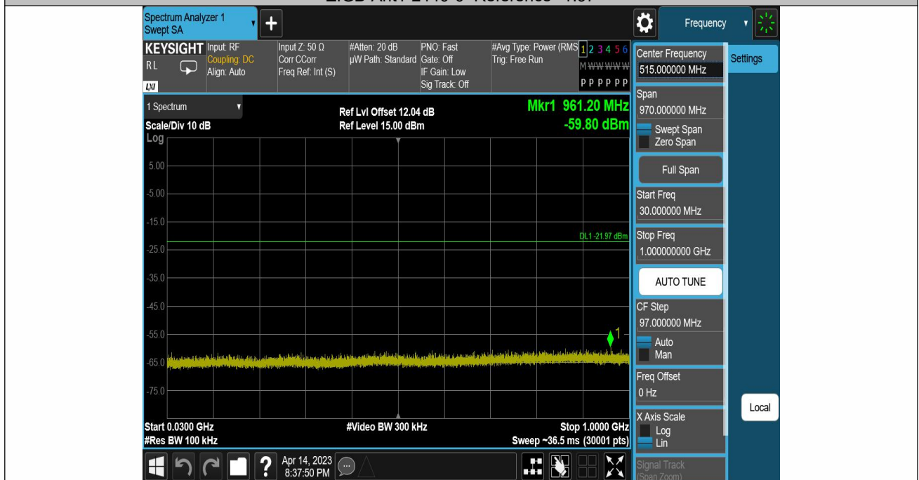
ZIGB-Ant1-2440-30~1000--1.97
