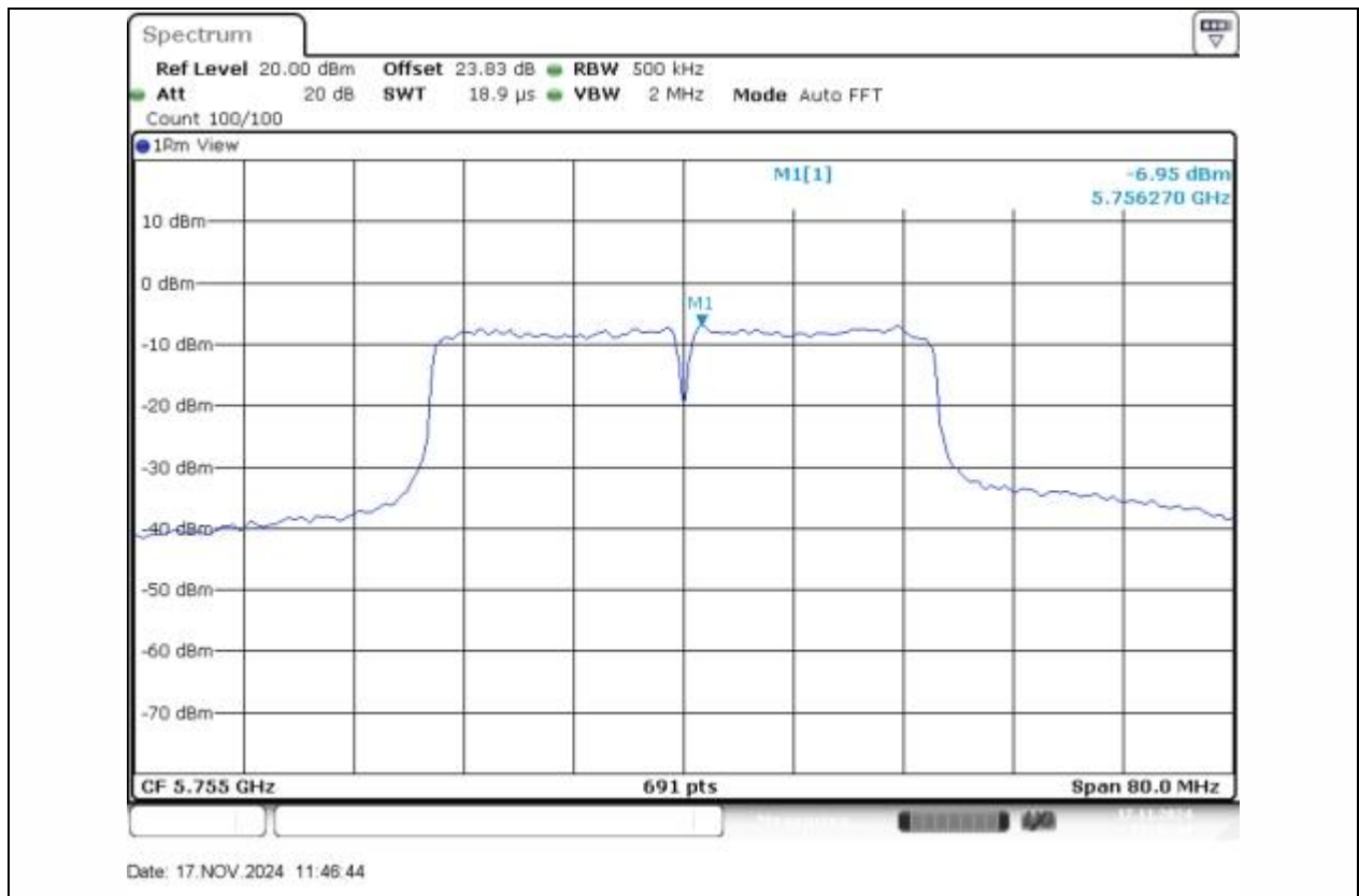
11N40SISO-Ant1-5755-PASS
