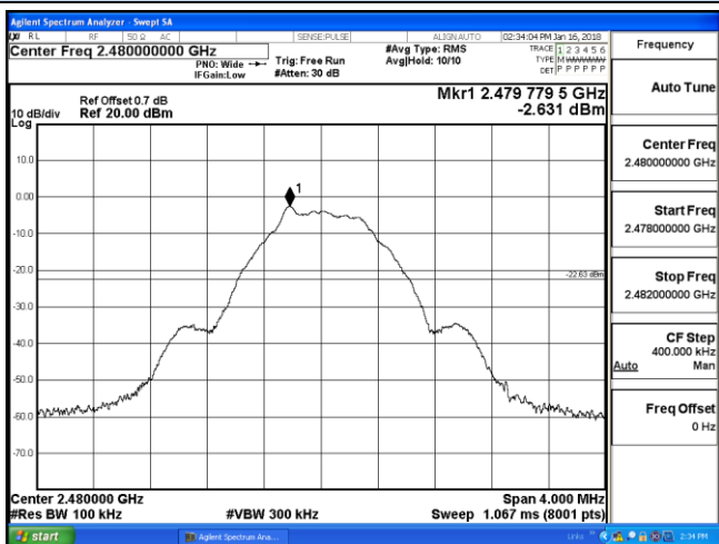
2480 MHz
