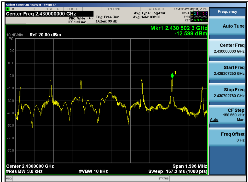
Test_Graph_SRD_ANT1_2430_GFSK_PSD
