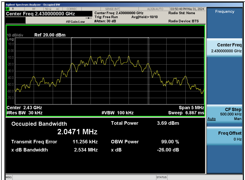
Test_Graph_SRD_ANT1_2430_GFSK_OBW
