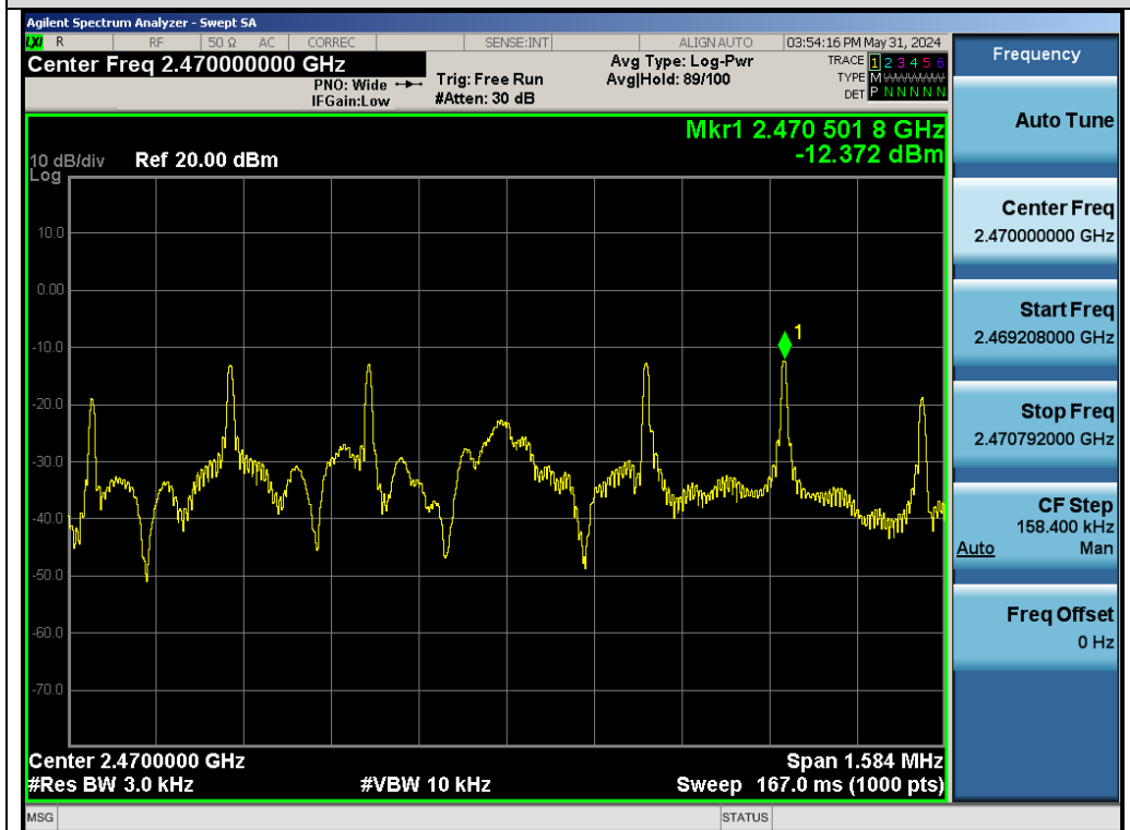
Test_Graph_SRD_ANT1_2470_GFSK_PSD
