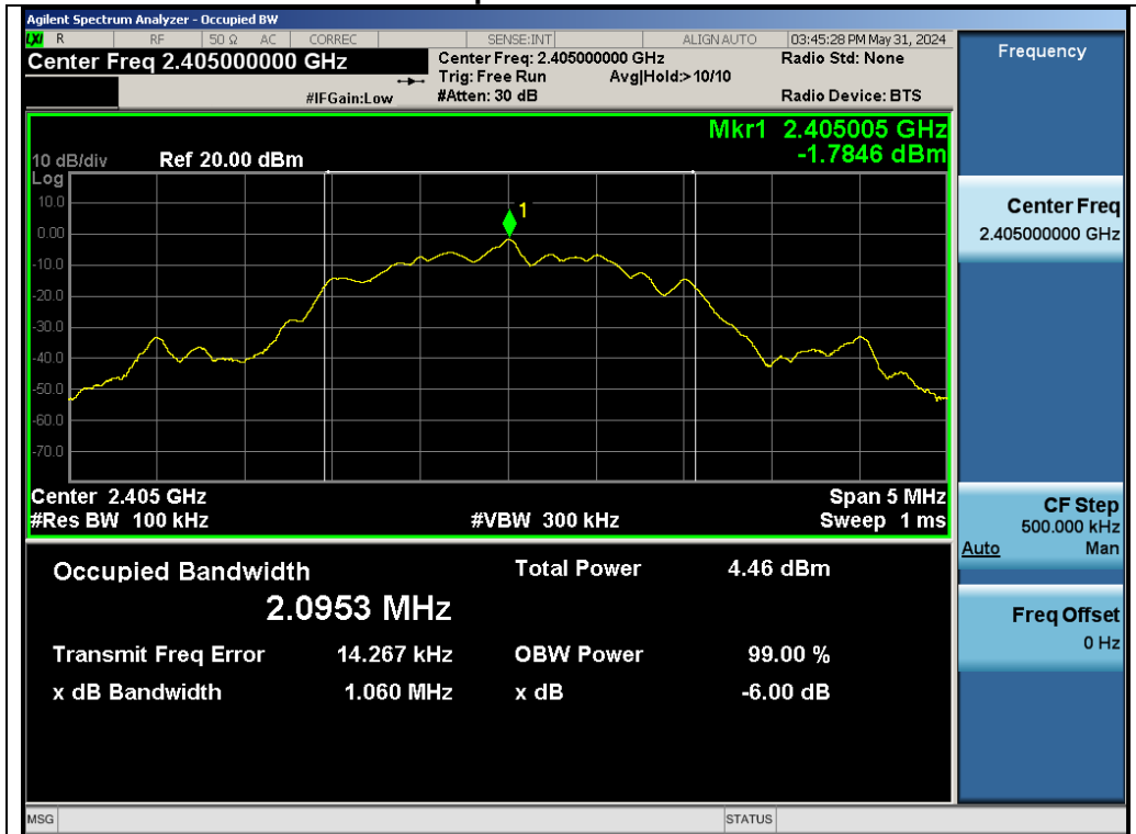
Test_Graph_SRD_ANT1_2405_GFSK_DTSBW
