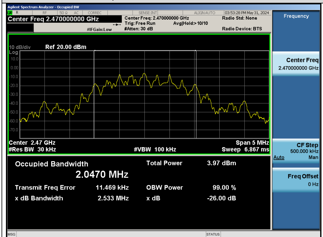
Test_Graph_SRD_ANT1_2470_GFSK_OBW
