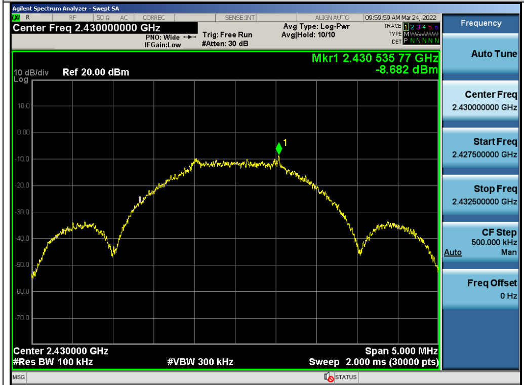
Test_Graph_GFSK_ANT1_2430_2Mbps_Reference Level
