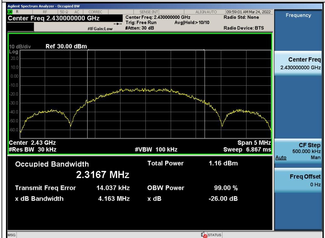
Test_Graph_GFSK_ANT1_2430_2Mbps_OBW
