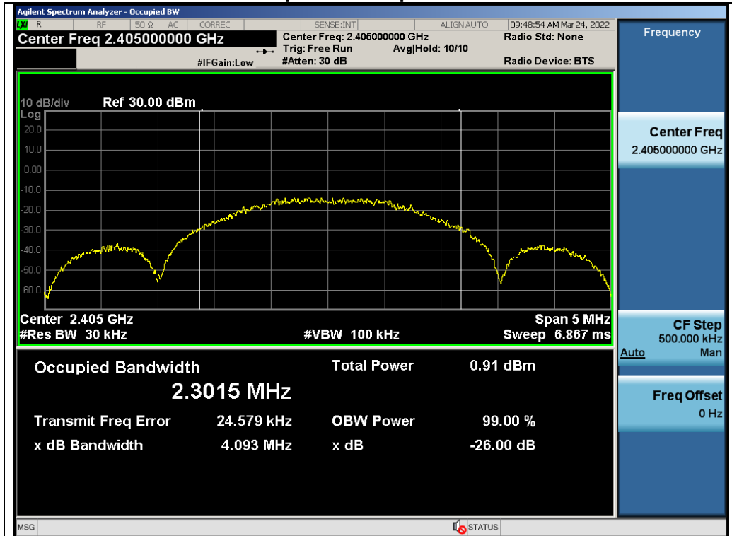
Test_Graph_GFSK_ANT1_2405_2Mbps_OBW
