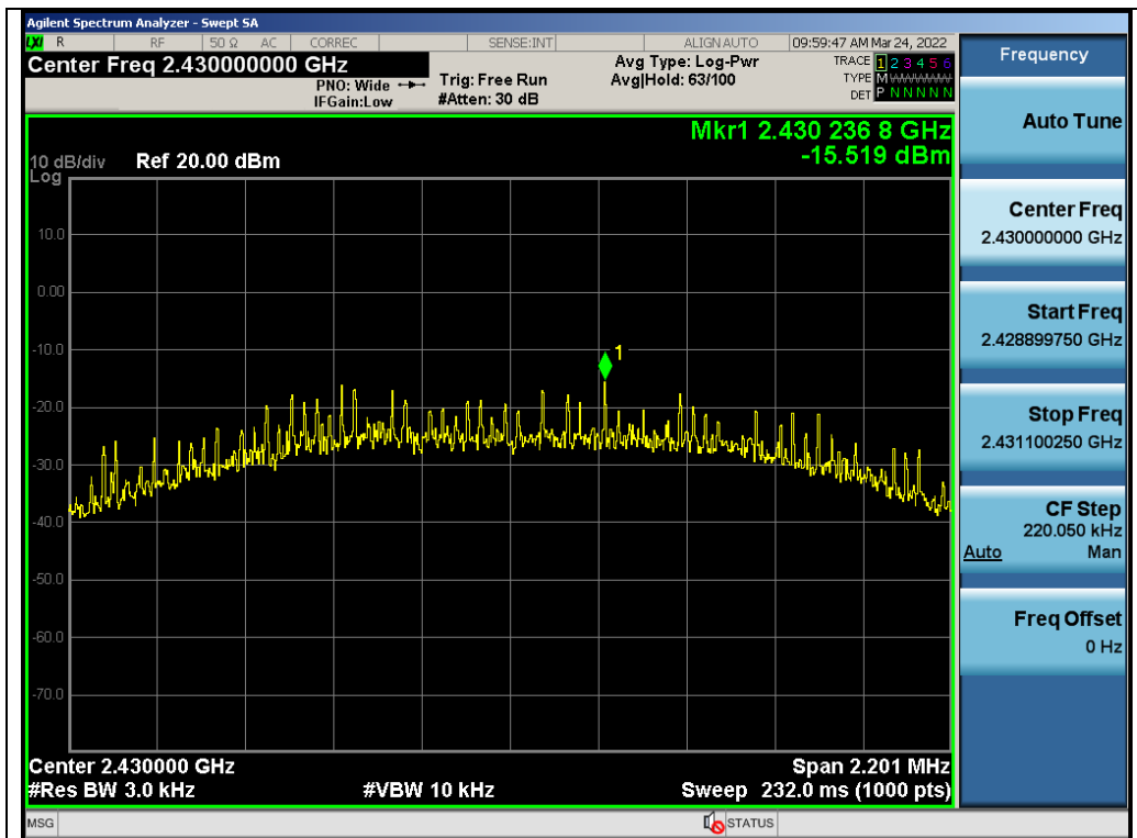
Test_Graph_GFSK_ANT1_2430_2Mbps_PSD
