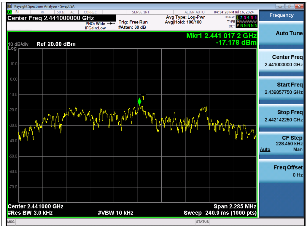
Test_Graph_2.4G_ANT1_2441_PSD
