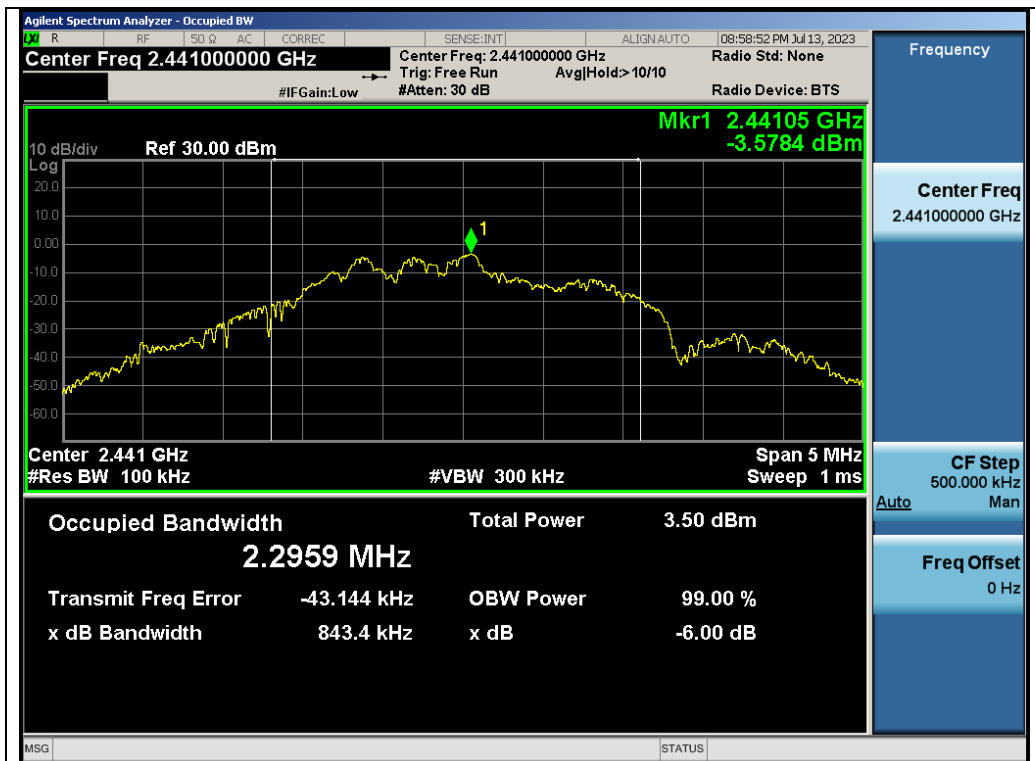
Test_Graph_2.4G_ANT1_2441_2Mbps_DTSBW
