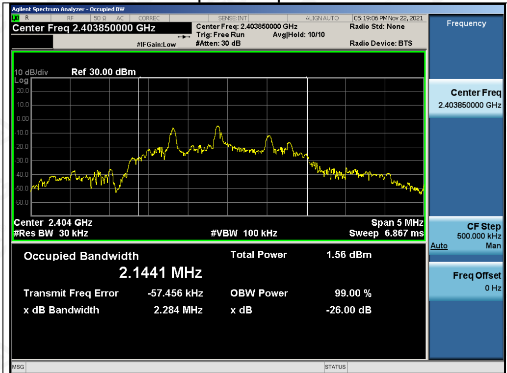
Test_Graph_ANT1_2403.85_OBW
