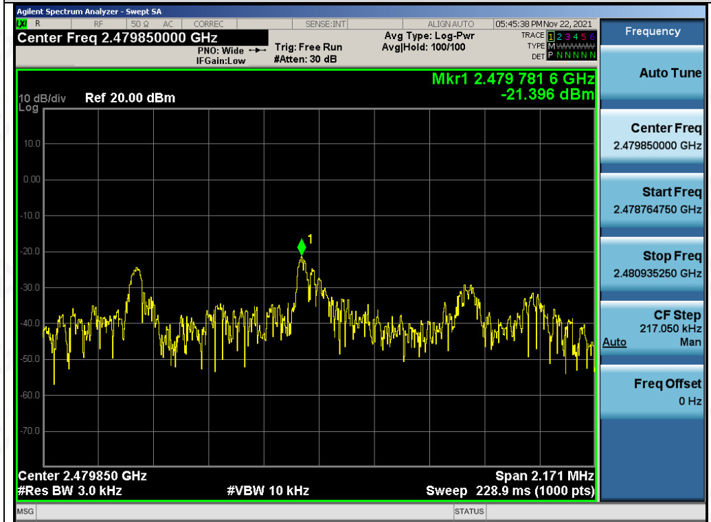
Test_Graph_LE2M_ANT1_2479.85_2Mbps_PSD
