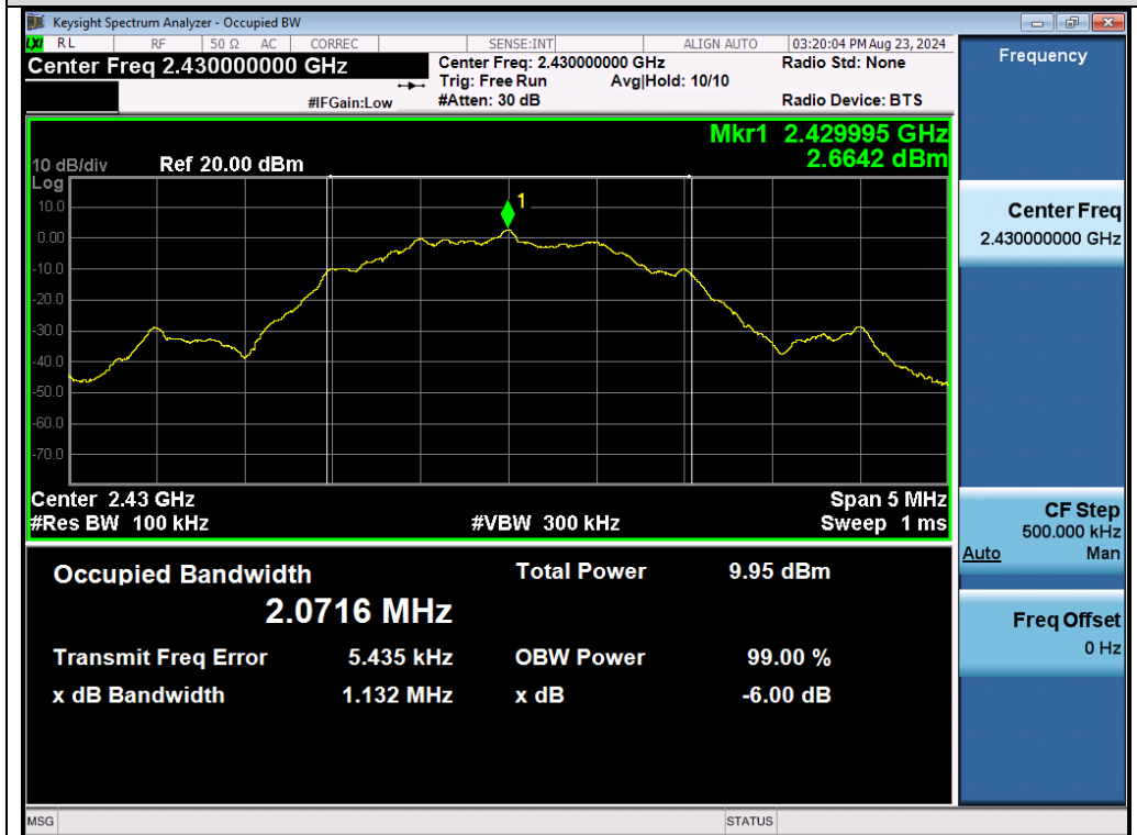
Test_Graph_GFSK_ANT1_2430_DTSBW
