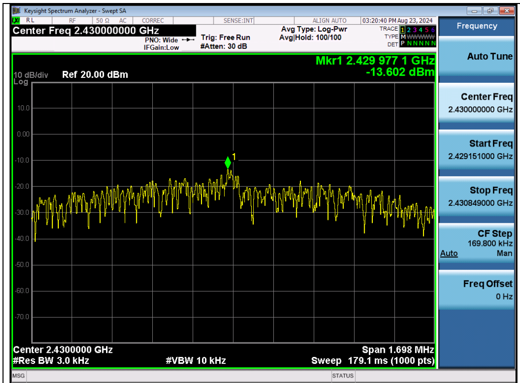
Test_Graph_GFSK_ANT1_2430_PSD
