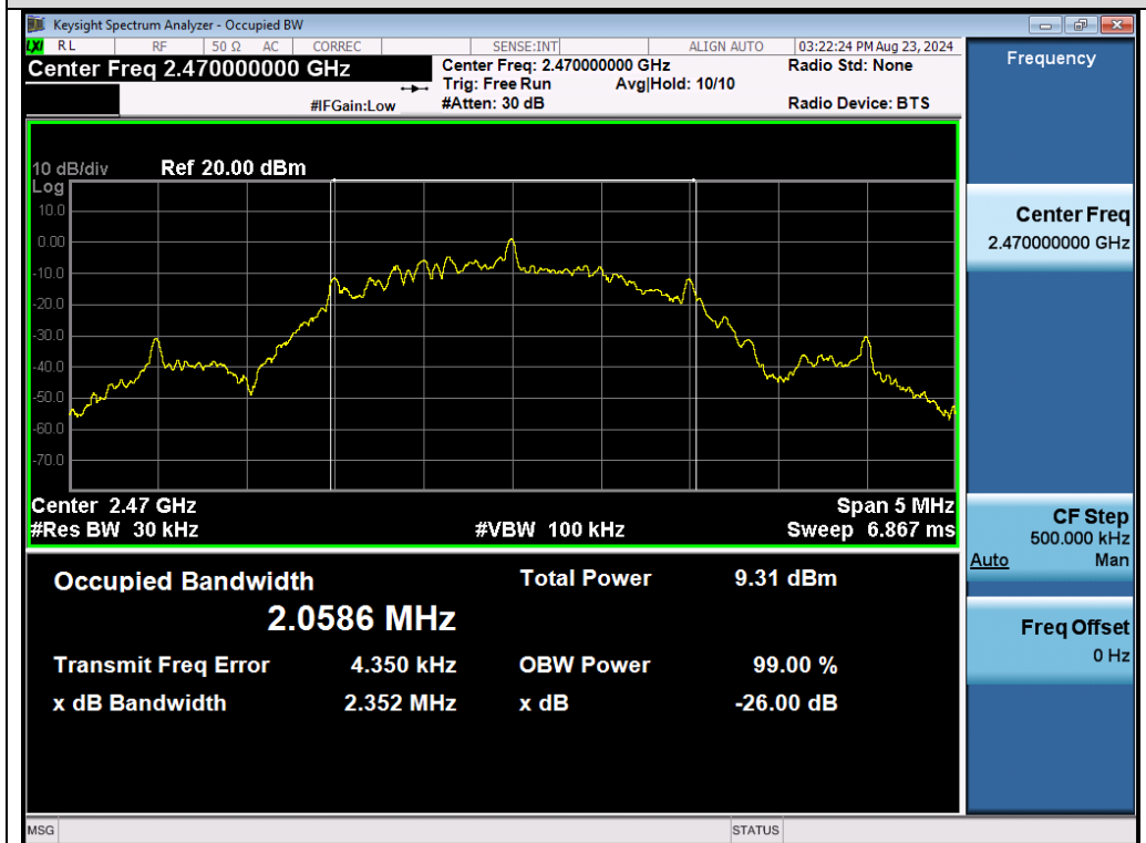
Test_Graph_GFSK_ANT1_2470_OBW
