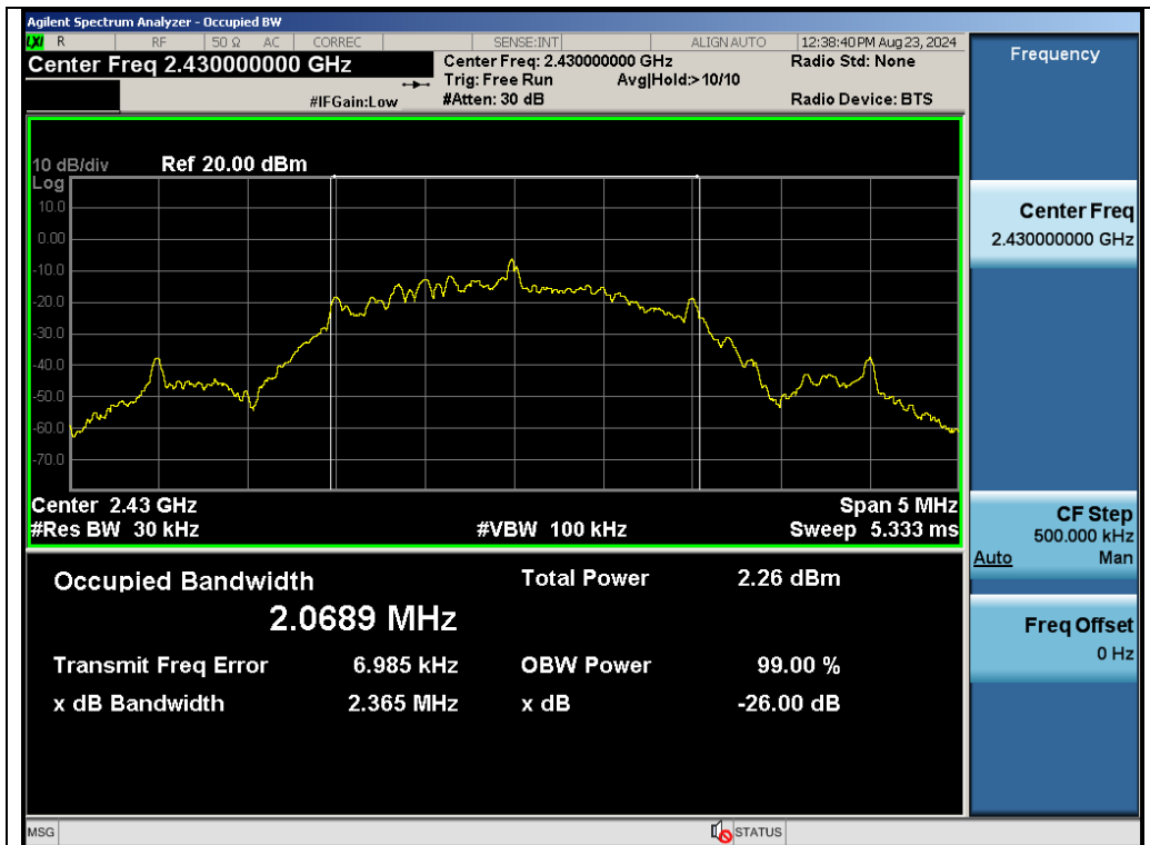
Test_Graph_GFSK_ANT1_2430_OBW
