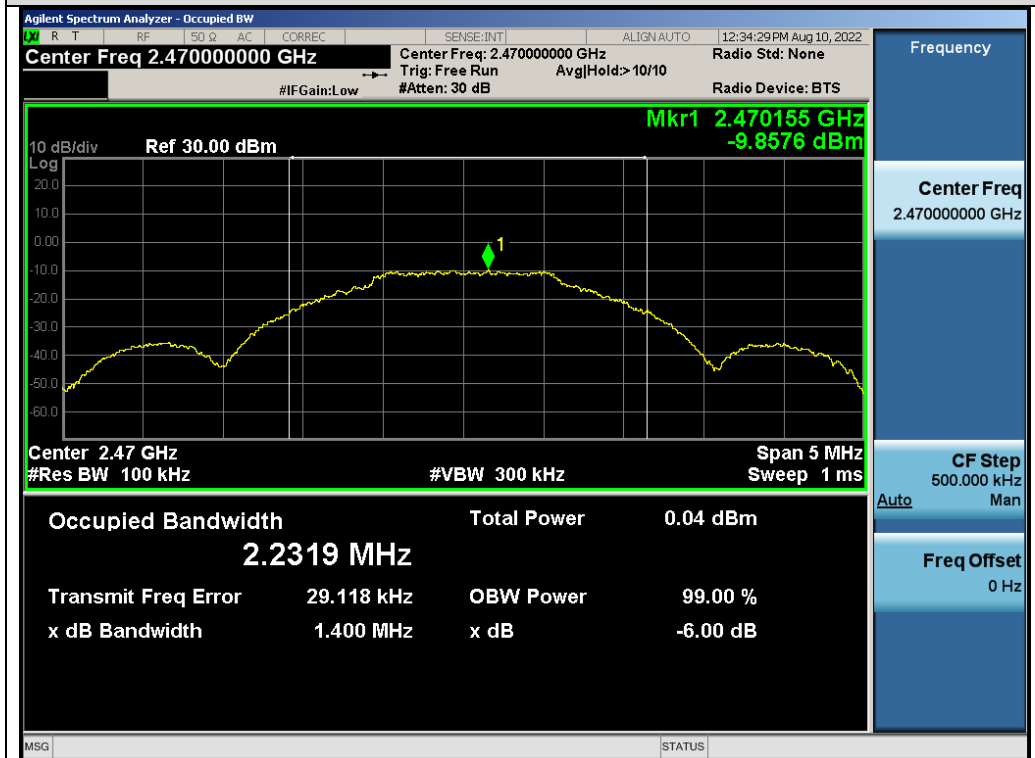
Test_Graph_GFSK_ANT1_2470_DTSBW
