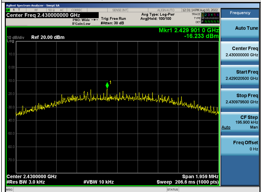
Test_Graph_GFSK_ANT1_2430_PSD
