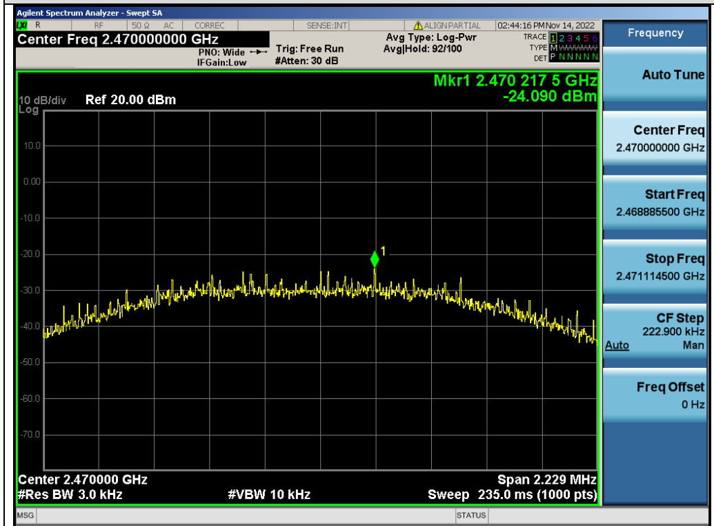
Test_Graph_GFSK_ANT1_2470_PSD
