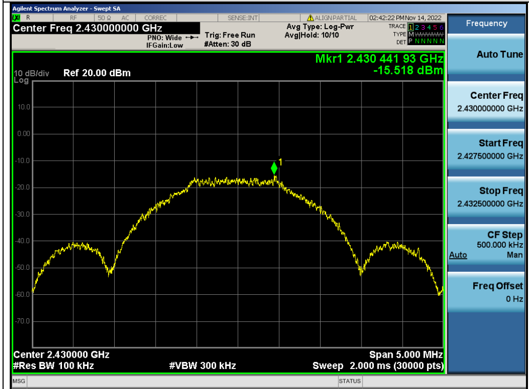
Test_Graph_GFSK_ANT1_2430_Reference Level
