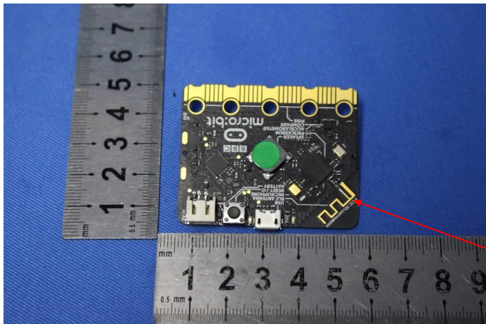
BLE antenna
