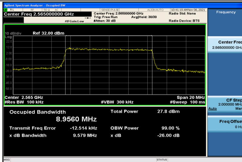
Band7-10MHz-QPSK-21400-50RB#0-8.9560
