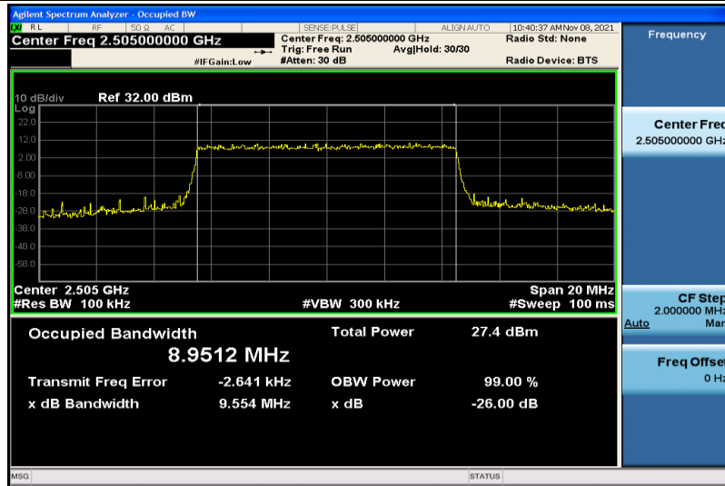
Band7-10MHz-QPSK-20800-50RB#0-8.9512
