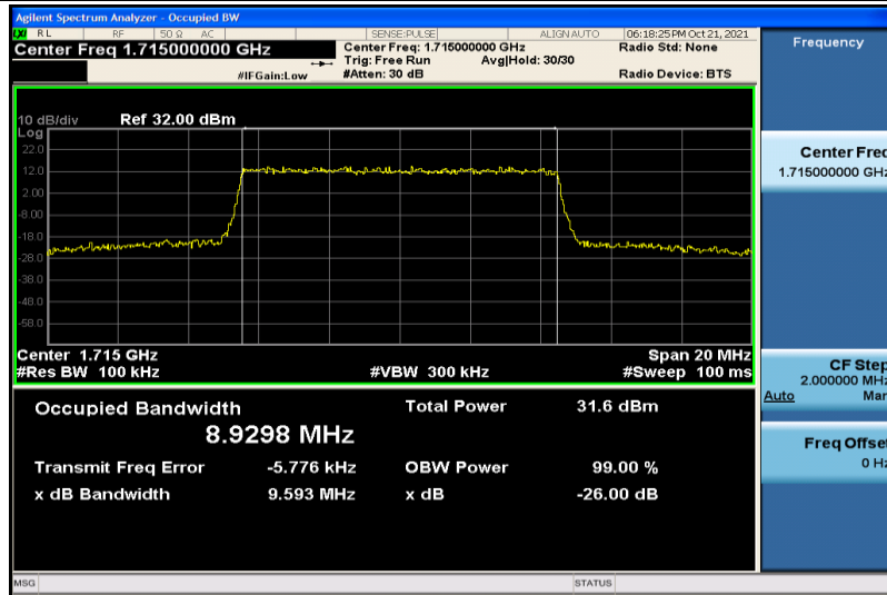
Band4-10MHz-QPSK-20000-50RB#0-8.9298
