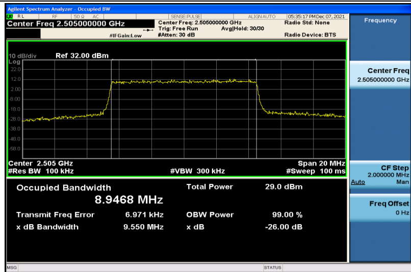
Band7-10MHz-QPSK-20800-50RB#0-8.9468
