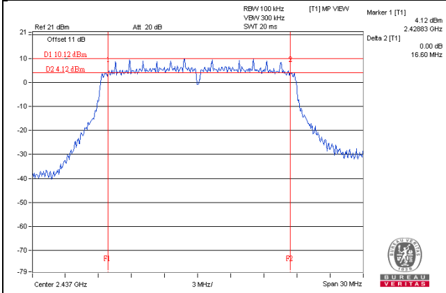
VHT20 / Chain 3 : CH6
