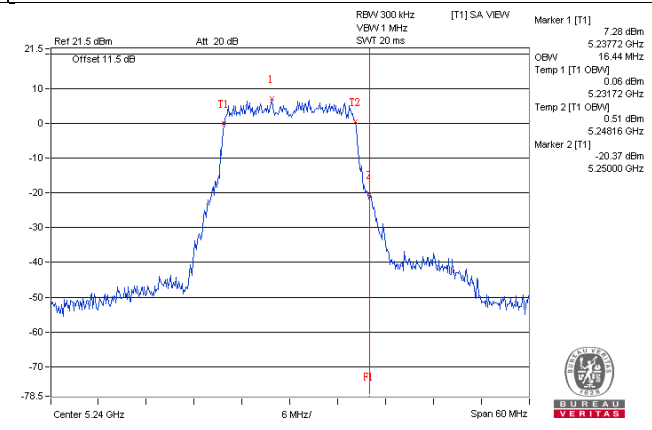
802.11a_Chain3 / CH48
