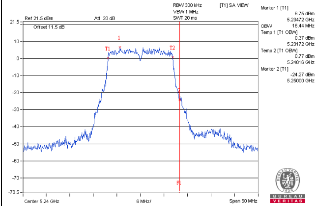
802.11a_Chain2 / CH48
