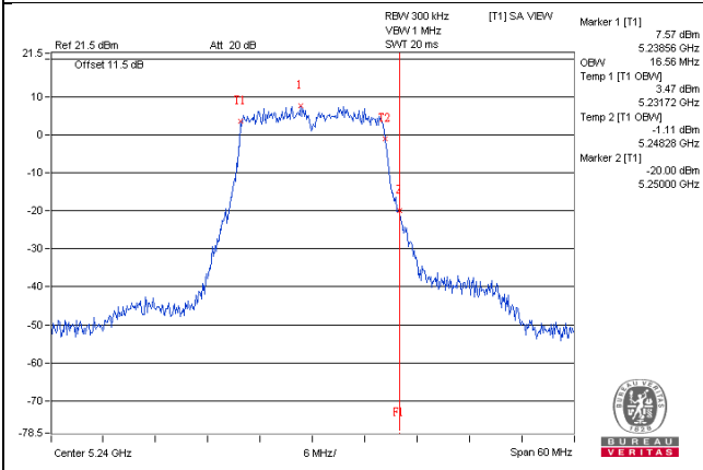
802.11a_Chain2 / CH48
