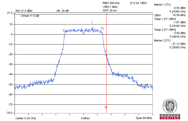
802.11a_Chain3 / CH48
