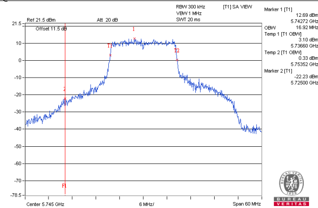
802.11a_Chain3 / CH149
