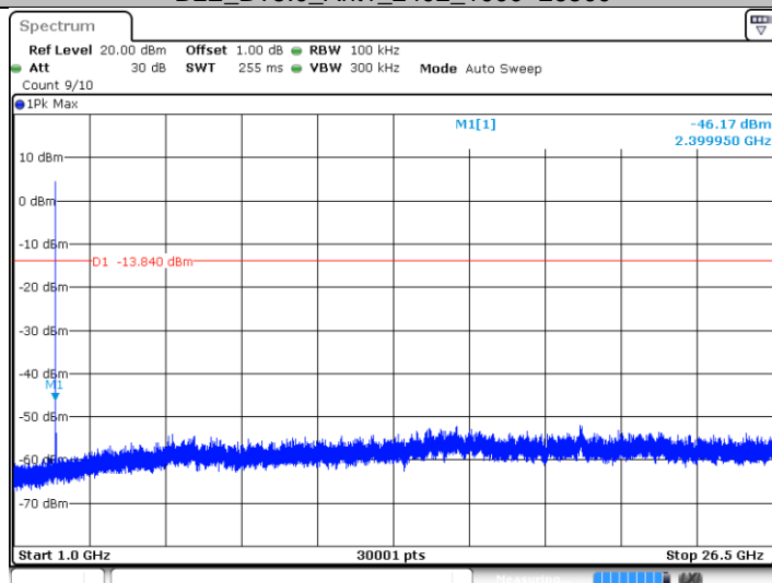
BLE_BT5.0_Ant1_2402_1000~26500
