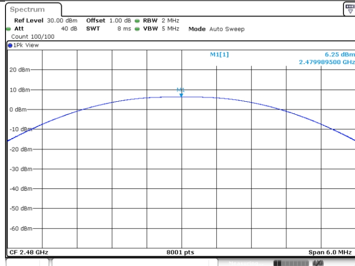
BLE_BT5.0_Ant1_2480
