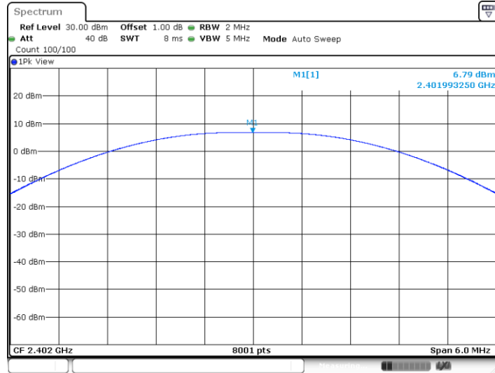
BLE_BT5.0_Ant1_2402
