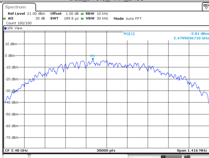
BLE_BT5.0_Ant1_2480
