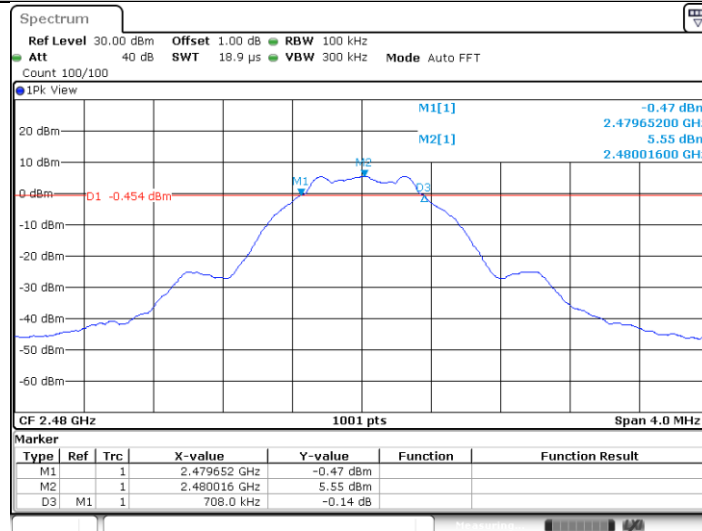
BLE_BT5.0_Ant1_2480
