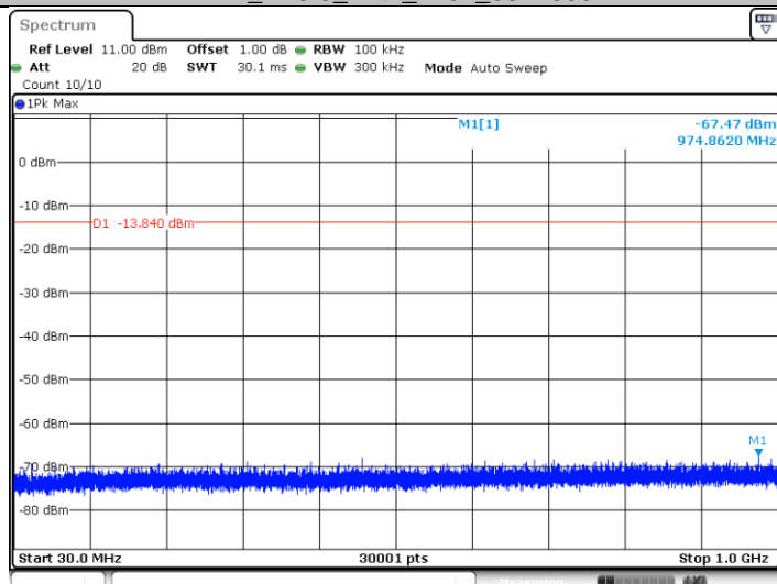
BLE_BT5.0_Ant1_2402_30~1000
