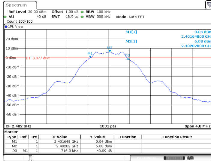
BLE_BT5.0_Ant1_2402
