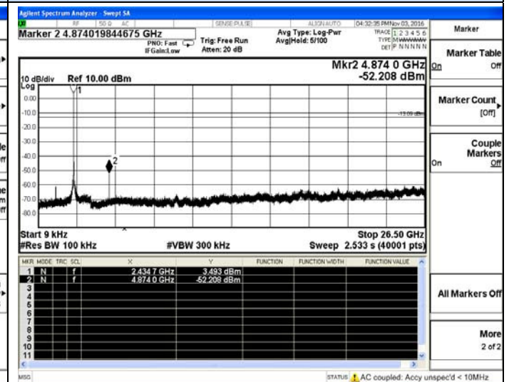
IEEE 802.11b-Middle channel
