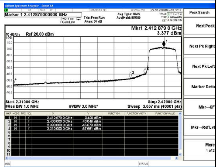
IEEE 802.11n(HT20)-Low channel(Average)
