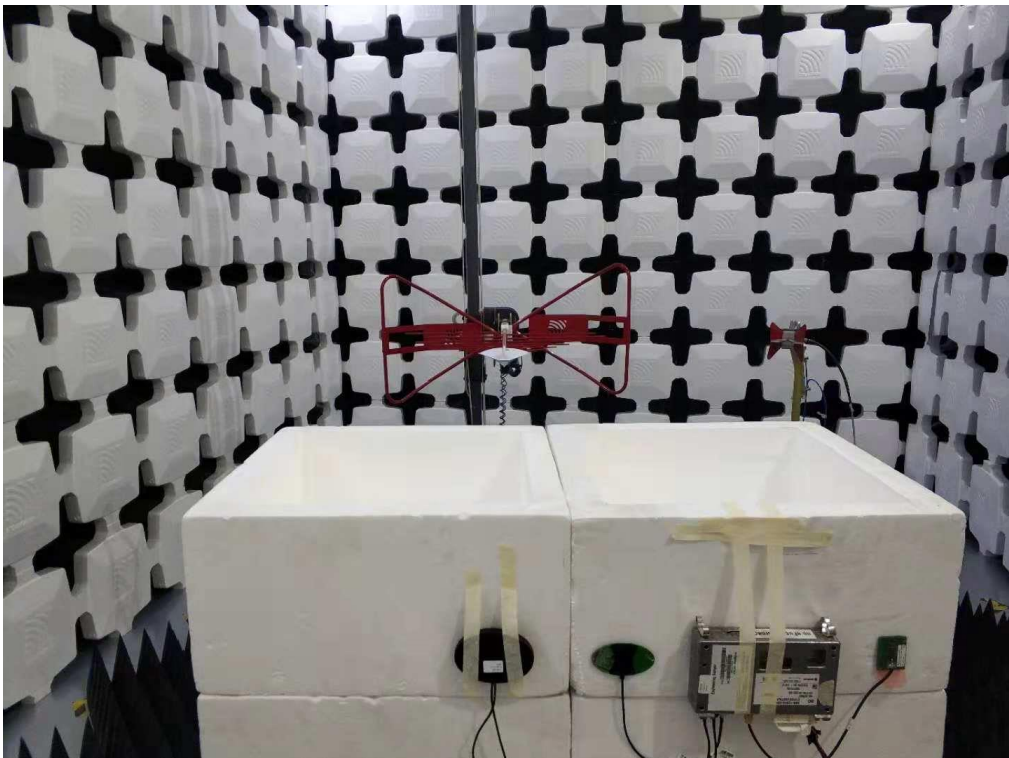
14. ERP/EIRP (EUT-V)
