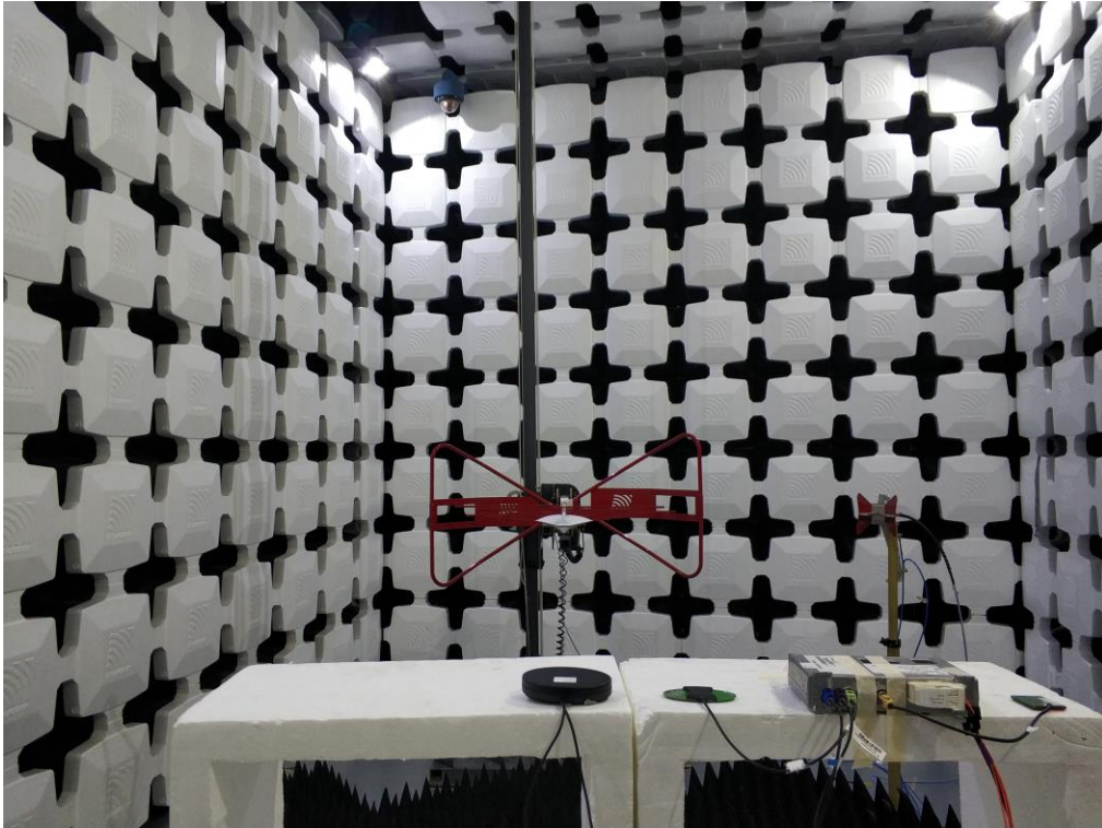
13. ERP/EIRP (EUT-H)
