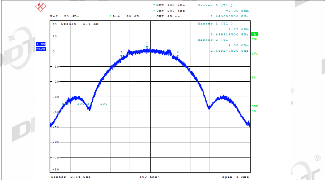
-6dB Bandwidth NVNT BLE 2M 2440MHz Ant1
