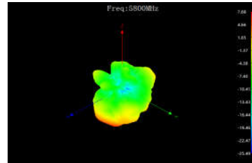
WiFi&BT Antenna
