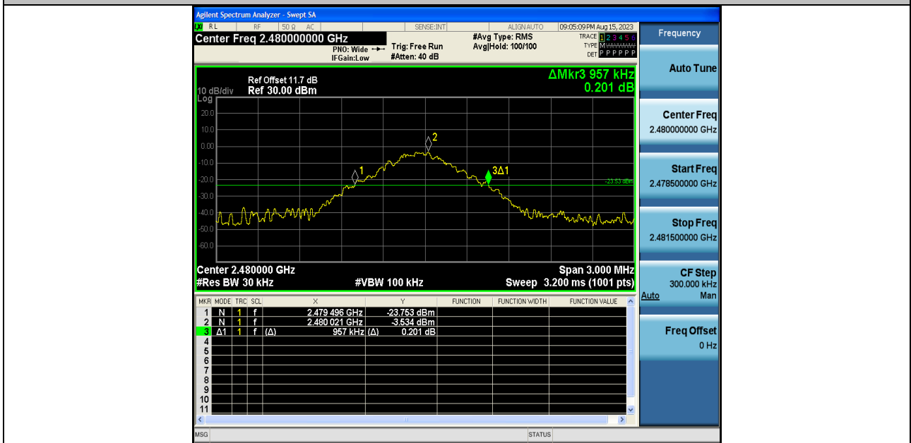
DH5-Ant1-2480
