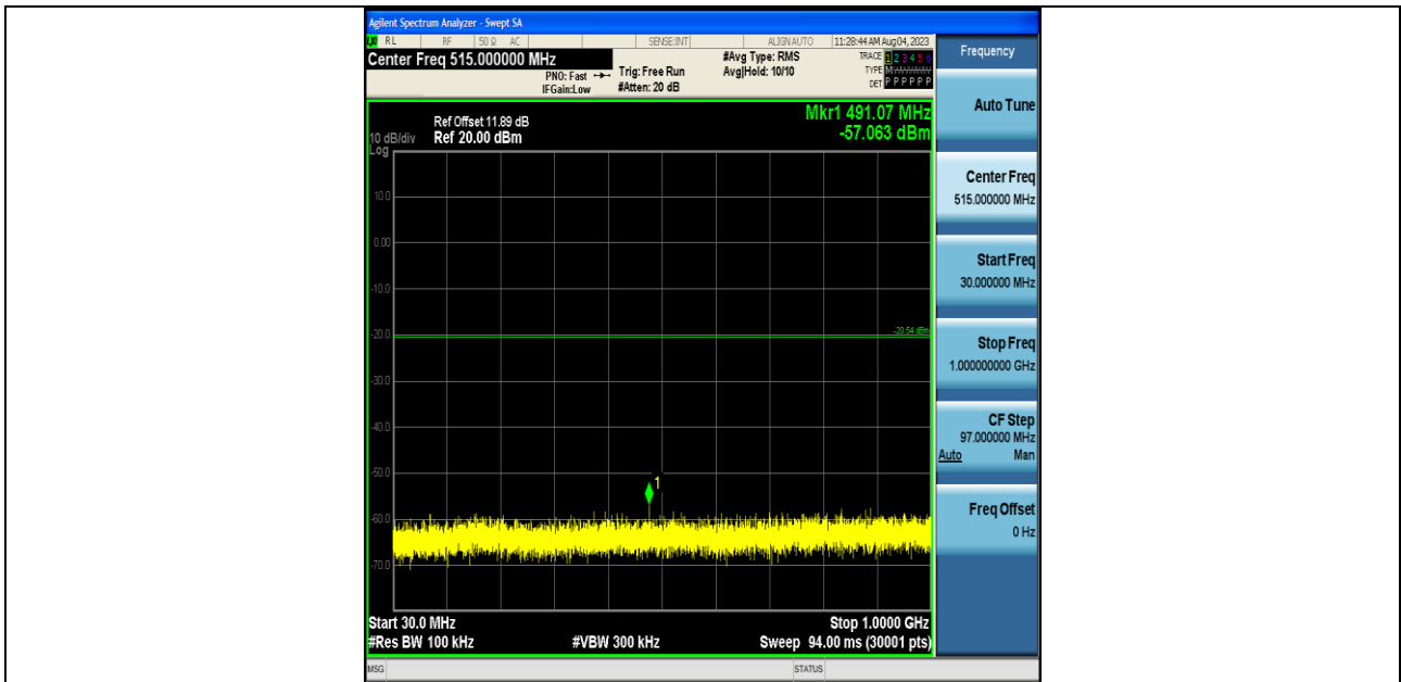
BLE_2M-Ant1-2402-30~1000-PASS
