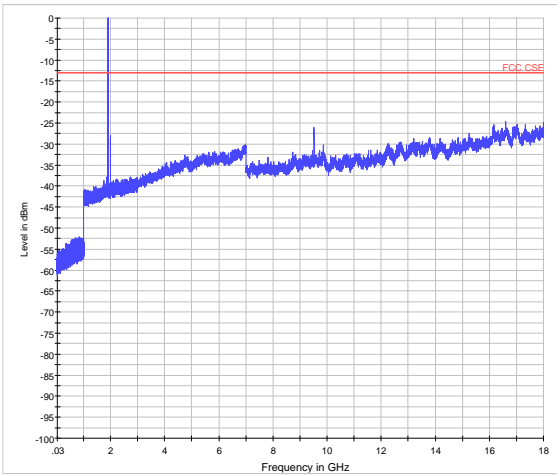
LTE Band 2 5MHz CH-High 30MHz~18GHz
