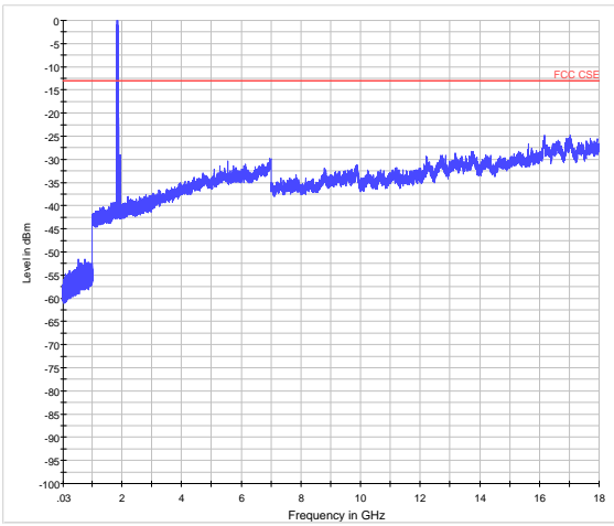
LTE Band 2 10MHz CH-Middle 30MHz~18GHz
