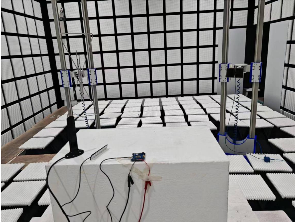
Pic1.RSE(30MHz-1GHz)
