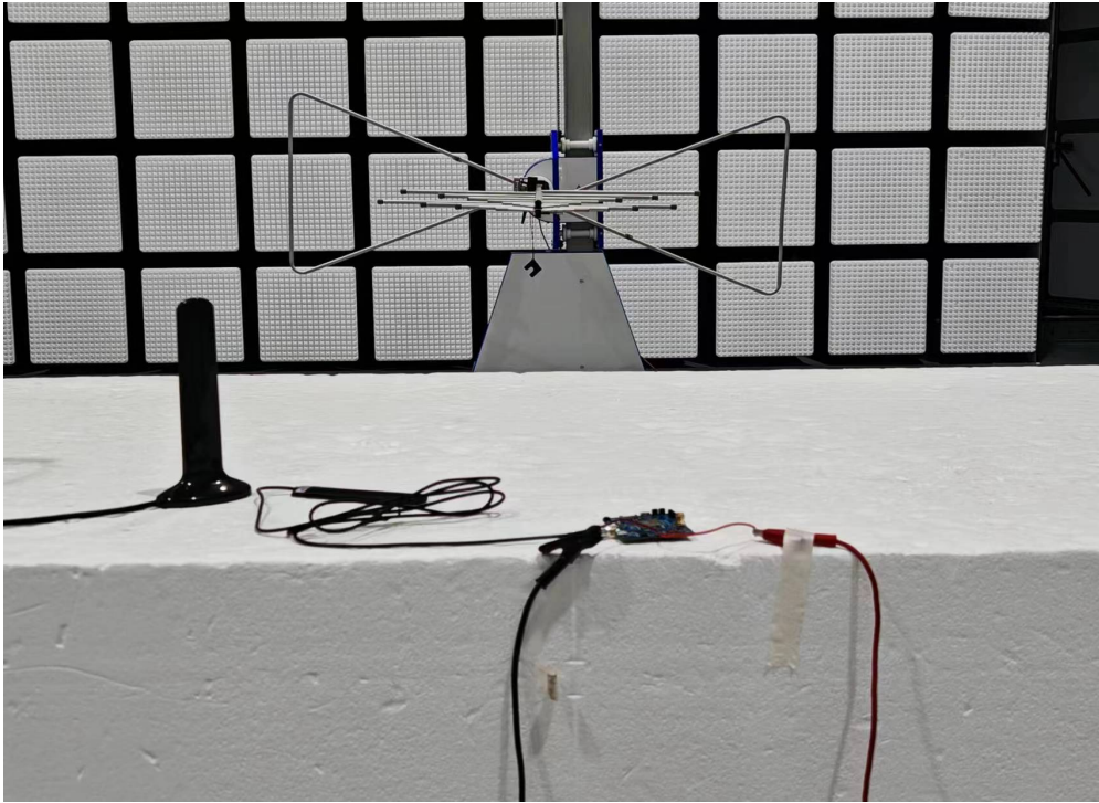
Pic1.RSE(30MHz-1GHz)
