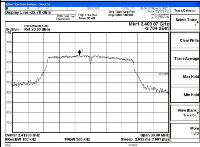
2397 – 2427 MHz
