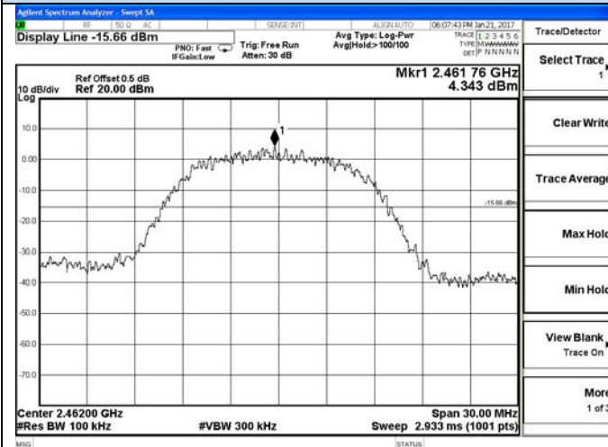
2447 – 2477 MHz
