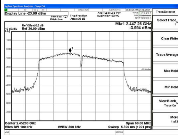
2422 – 2482 MHz
