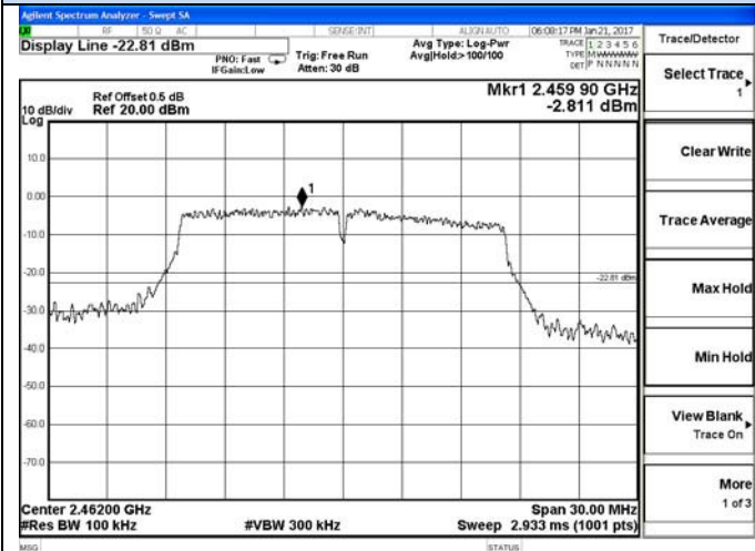
2447 – 2477 MHz
