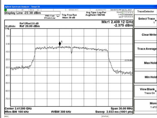
2397 – 2427 MHz
