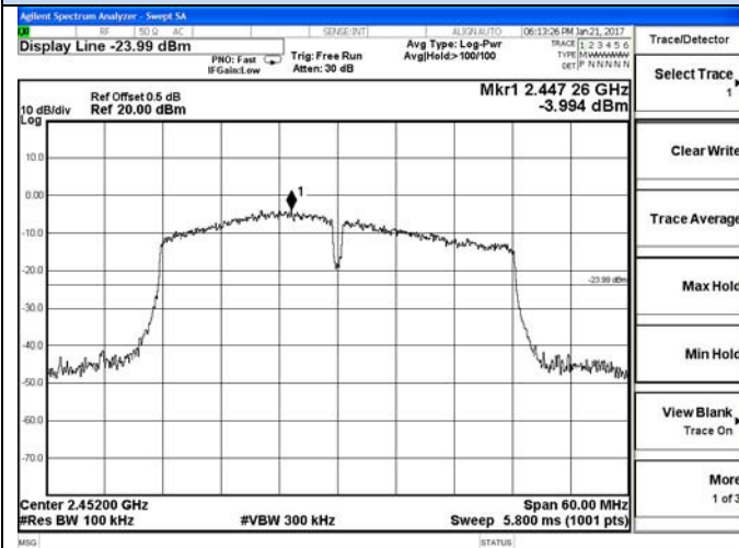
2422 – 2482 MHz
