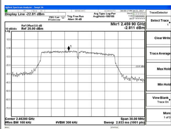
2447 – 2477 MHz
