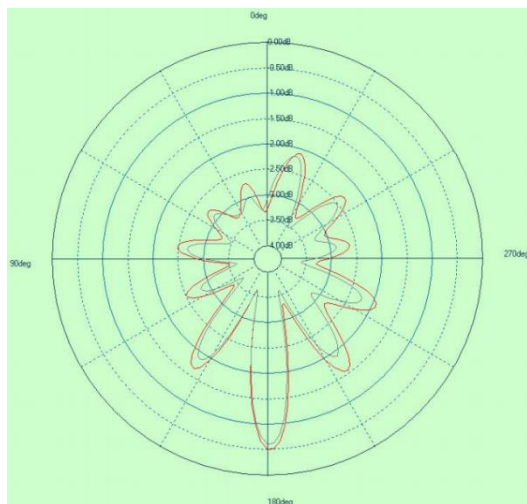
Theta=90°
