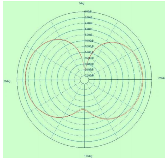
Phi=90°
