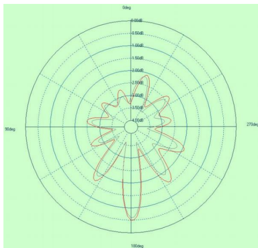
Theta=90°
