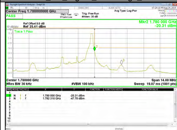
QPSK_3M_Higher_Band edge_1-RB
