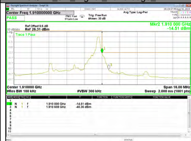
16QAM_5M_Higher_Band edge_1-RB
