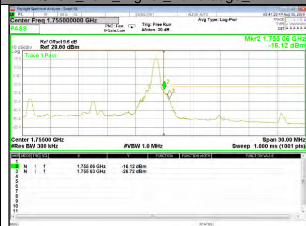
QPSK_15M_Higher_Band edge_1-RB
