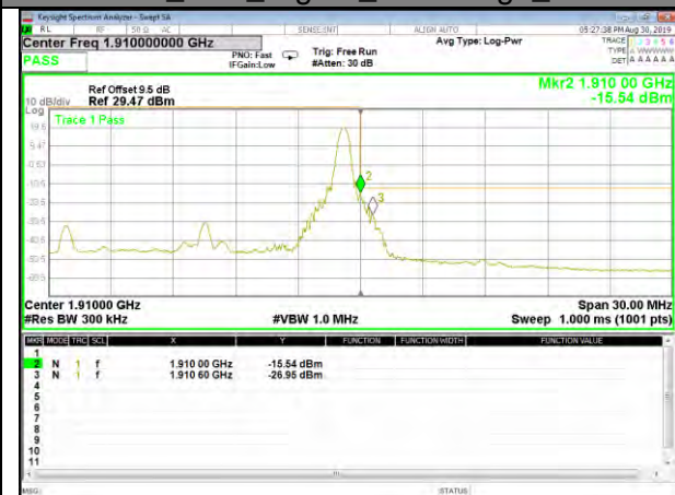
QPSK_15M_Higher_Band edge_1-RB
