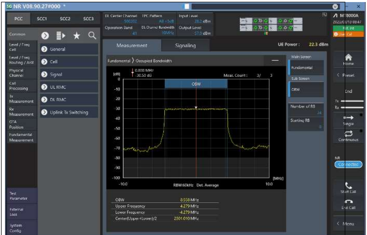
n41_10MHz_30kHz_500202_DFT-s-OFDM PI/2 BPSK^Outer_Full
