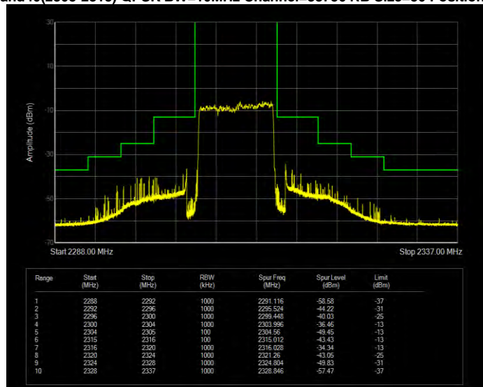
Band4(2305-2315) QPSK BW=10MHz Channel=38750 RB Size=50 Position=#0
