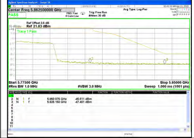
W58_11ac80_Band edge_Right
