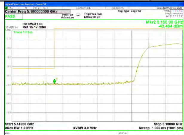
W52_11ac20_Lower_Band edge
