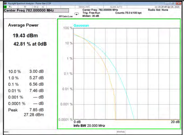
B13_50_Q16_Middle_
