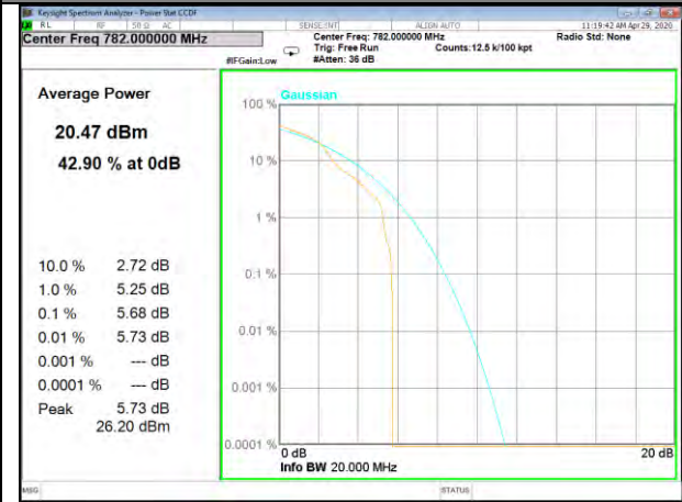
B13_1_Q16_Middle_
