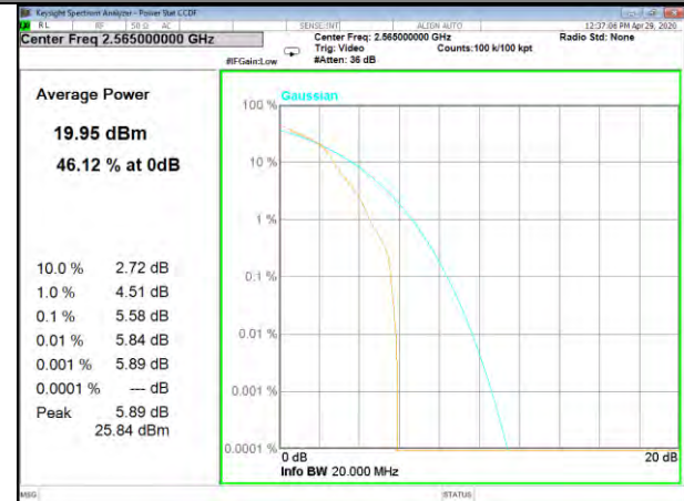
B41_1_QPSK_Middle_
