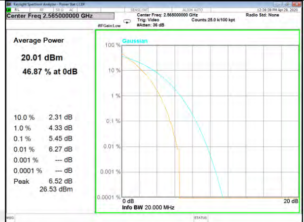
B41_100_Q16_Lower_
