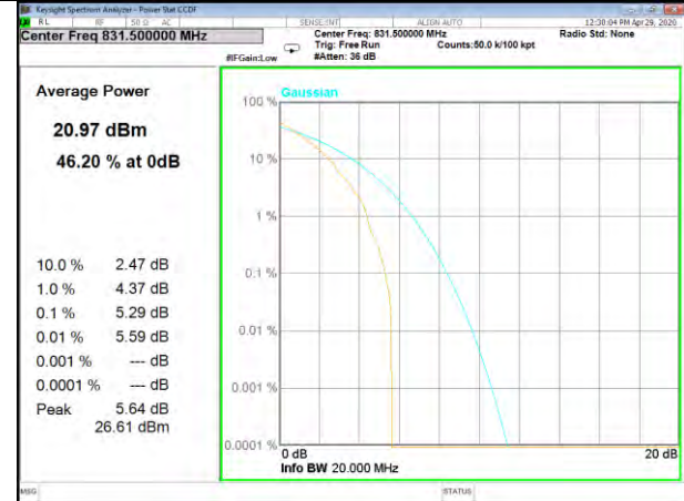
B26_1_Q16_Lower
