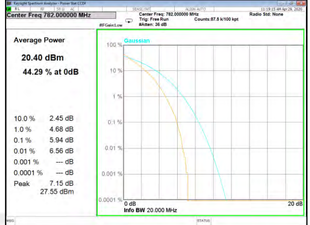
B13_50_Q16_Middle_
