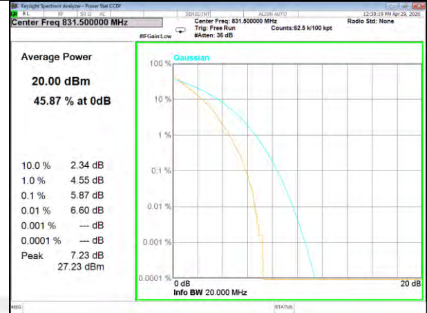
B26_50_Q16_Lower
