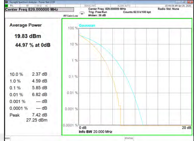
B5_50_Q16_Lower_
