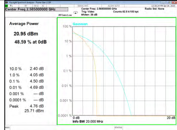
B41_1_Q16_Lower_
