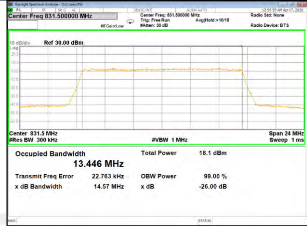
B26_Q16_15M_Mid_26BW-99%
