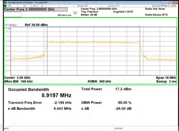
B41_Q16_10M_Mid_26BW-99%
