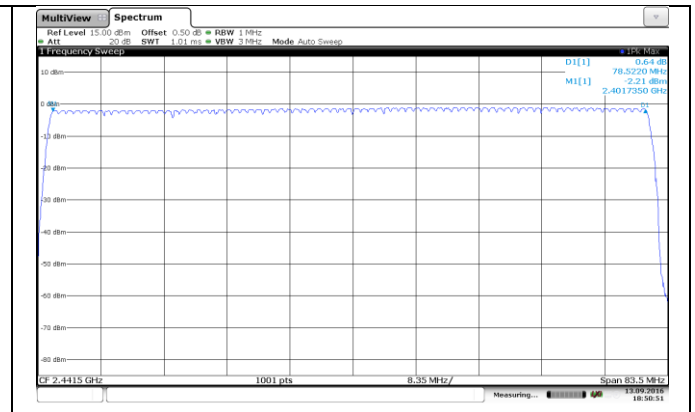
\pi/4 DQPSK
