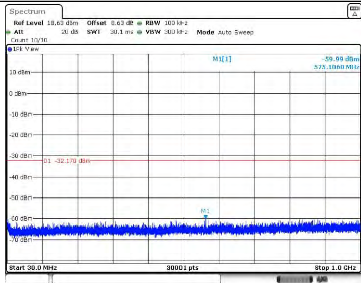
11AX40SISO_Ant1_2437_30~1000
