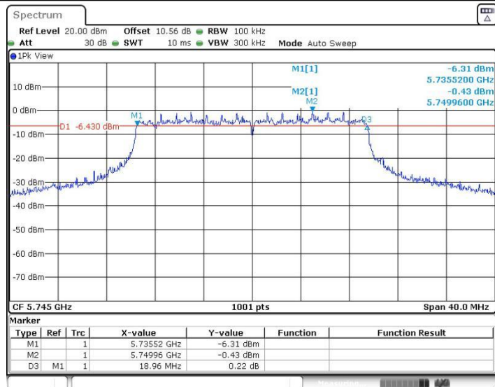
11AX20SISO_Ant1_5745
