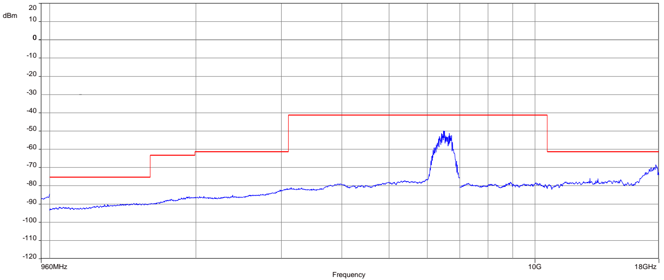
Plot 9: EUT2, 15.250 (d) (1), 960 MHz – 18 GHz
