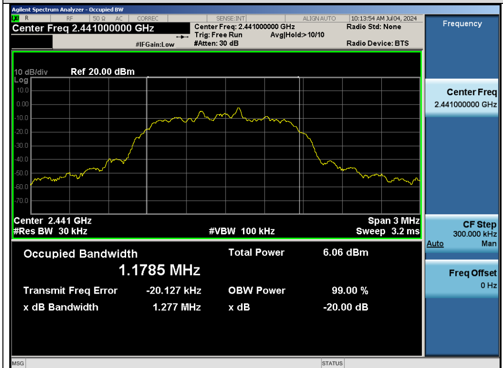
Test_Graph_EDR_ANT1_2441_2Mbps_OBW
