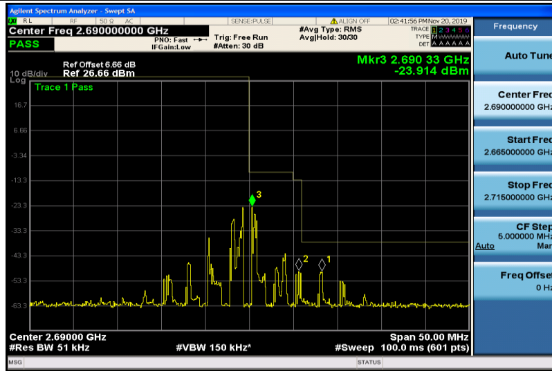
Band41-5MHz-16QAM-41565-1RB#24
