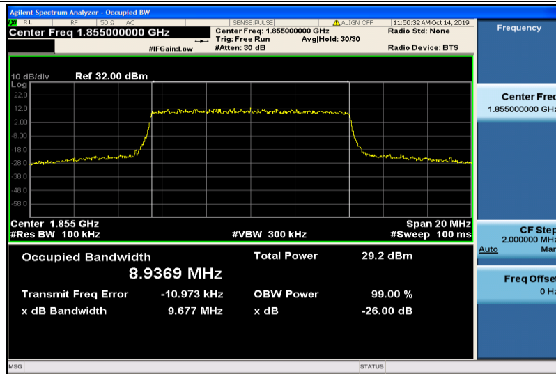
Band2-10MHz-QPSK-18650-50RB#0-8.9369
