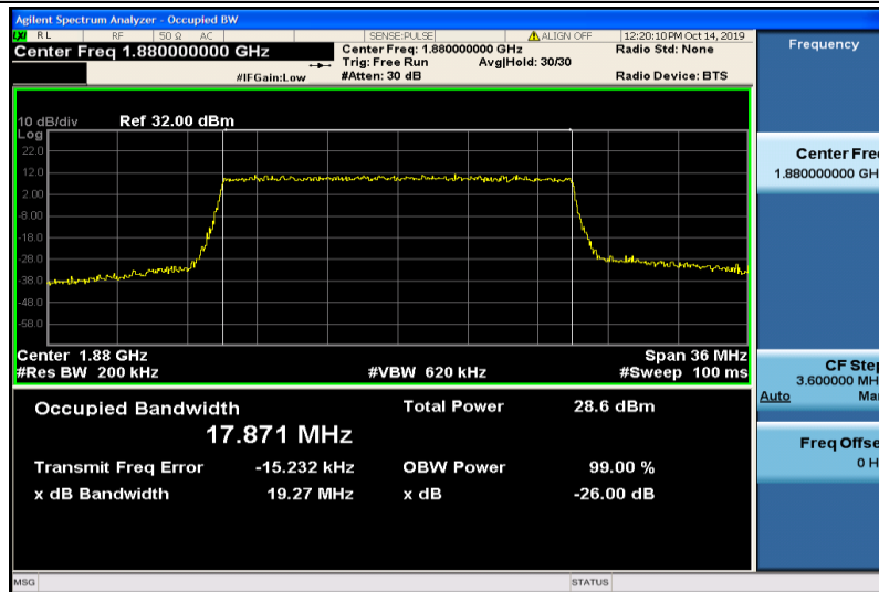
Band2-20MHz-16QAM-18900-100RB#0-17.871
