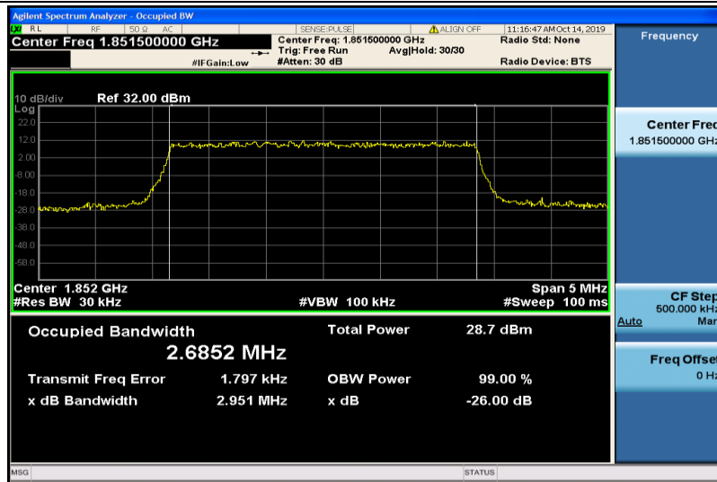
Band2-3MHz-QPSK-18615-15RB#0-2.6852
