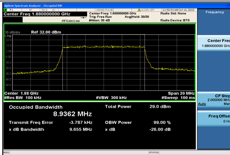
Band2-10MHz-QPSK-18900-50RB#0-8.9362
