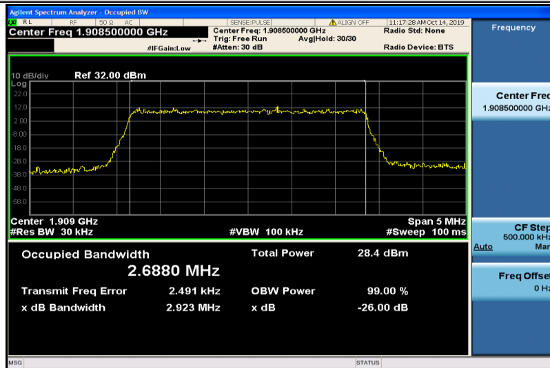
Band2-3MHz-QPSK-19185-15RB#0-2.6880
