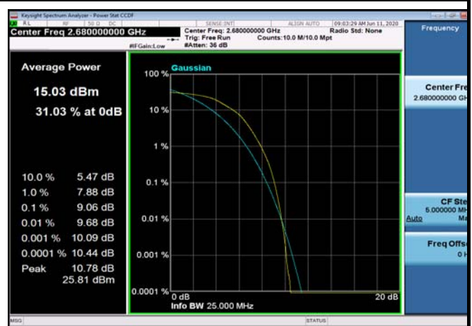
TDD41_HighRange_20MHz_2680_fullRB_Q16
