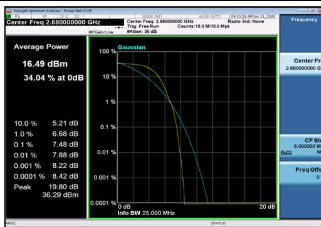
TDD41_HighRange_20MHz_2680_OneRB_high_Q16
