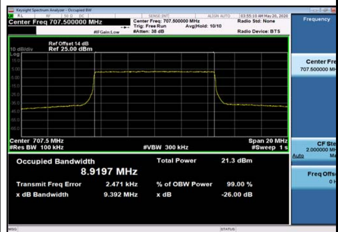
FDD12_MidRange_10_707.5_Q16
