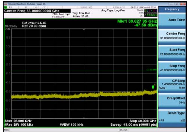
U-NII-2a ,Plot 2,26000MHz~40000MHz-80 2.11n(20MHz),5320MHz
