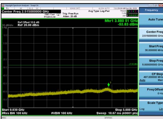
U-NII-2a ,Plot 2,30MHz~5000MHz-802.11 n(20MHz),5300MHz
