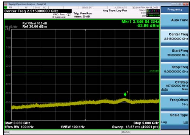
U-NII-2a ,Plot 2,30MHz~5000MHz-802.11 ac(20MHz),5320MHz
