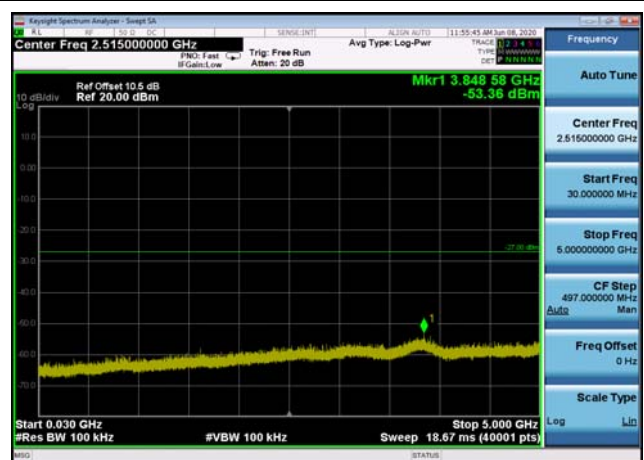
U-NII-2a ,Plot 2,30MHz~5000MHz-802.11 n(20MHz),5320MHz
