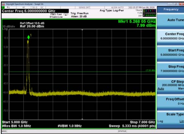
U-NII-2a ,Plot 3,5000MHz~7000MHz-802. 11ac(20MHz),5260MHz
