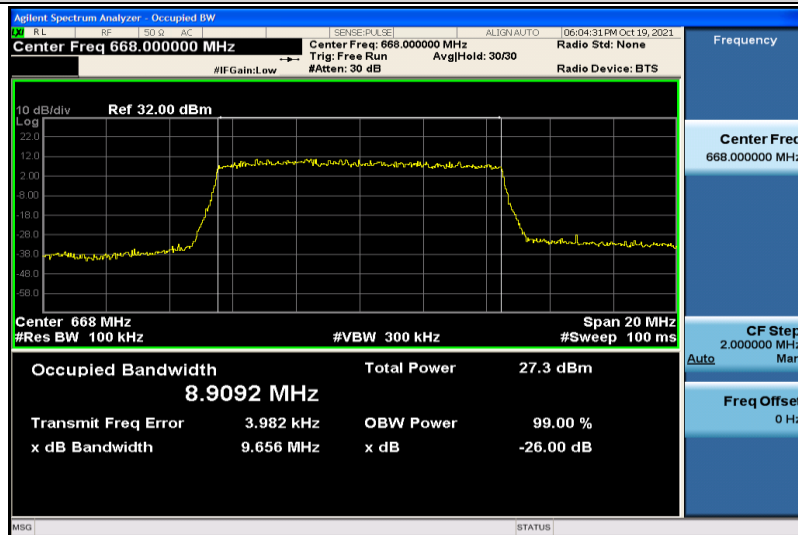
Band71-10MHz-QPSK-133172-50RB#0-8.9092
