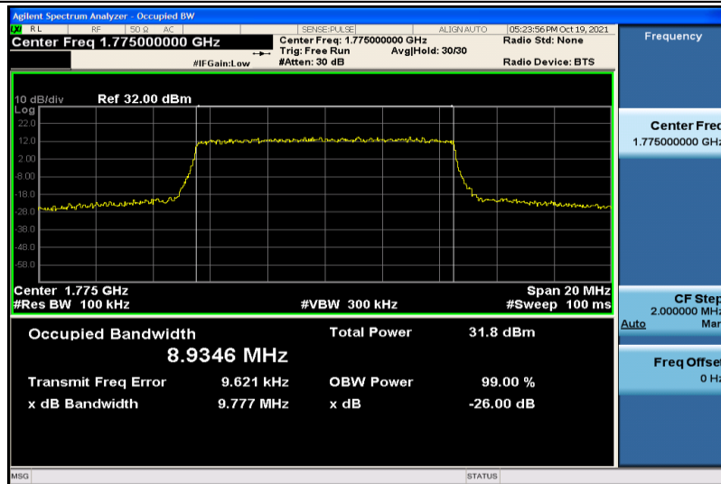
Band66-10MHz-QPSK-132622-50RB#0-8.9346
