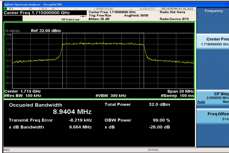
Band4-10MHz-QPSK-20000-50RB#0-8.9404
