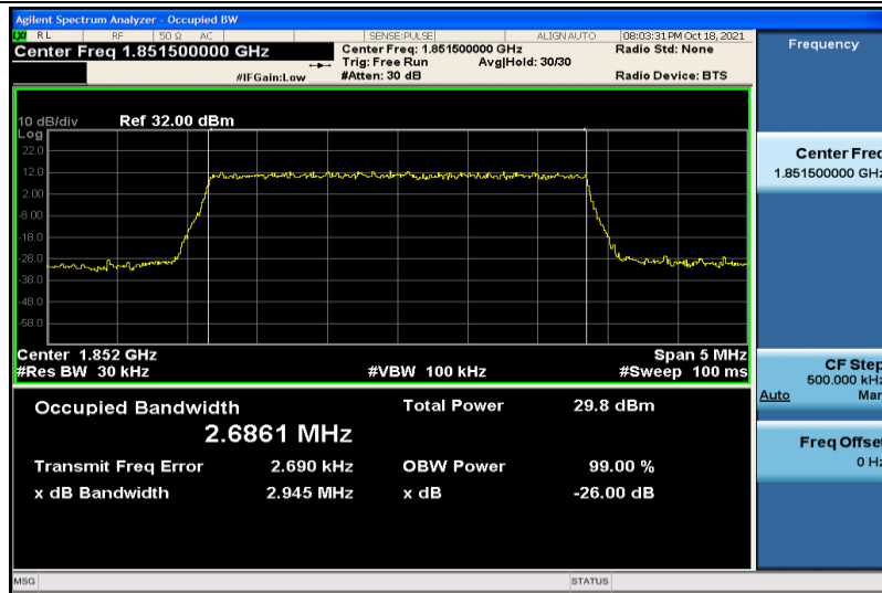
Band2-3MHz-QPSK-18615-15RB#0-2.6861
