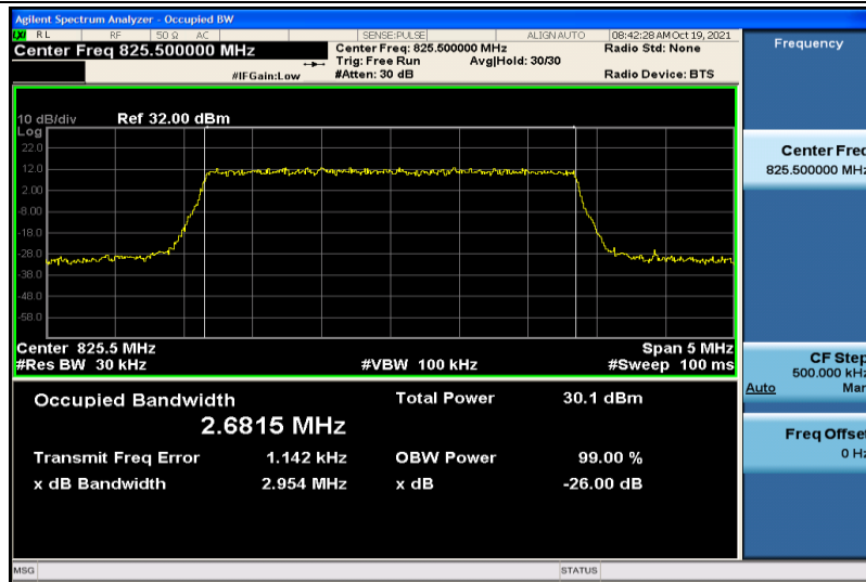
Band5-3MHz-QPSK-20415-15RB#0-2.6815
