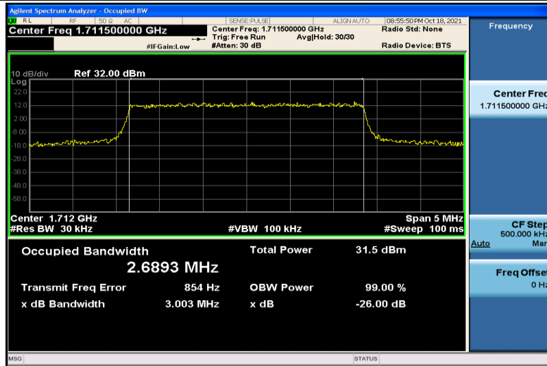
Band4-3MHz-QPSK-19965-15RB#0-2.6893
