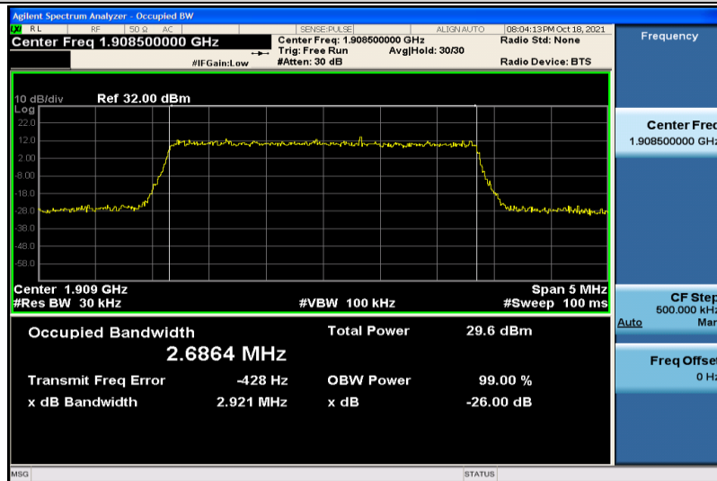
Band2-3MHz-QPSK-19185-15RB#0-2.6864
