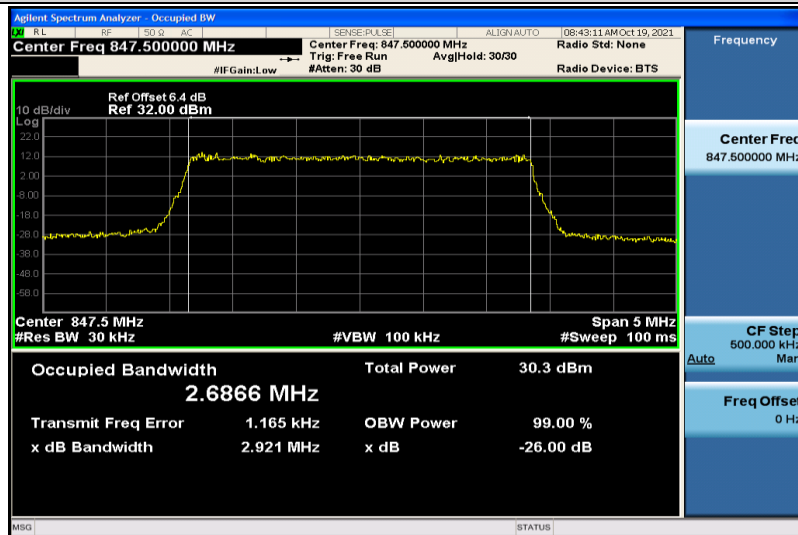
Band5-3MHz-QPSK-20635-15RB#0-2.6866
