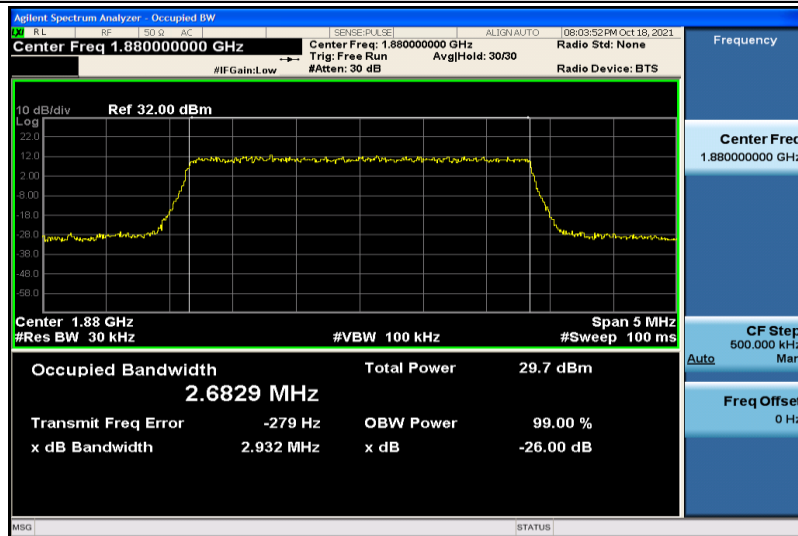
Band2-3MHz-QPSK-18900-15RB#0-2.6829
