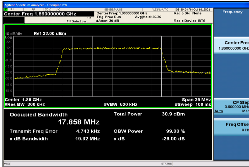
Band2-20MHz-QPSK-18700-100RB#0-17.858
