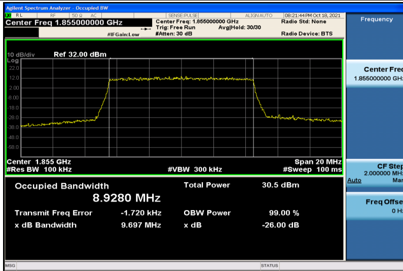
Band2-10MHz-QPSK-18650-50RB#0-8.9280
