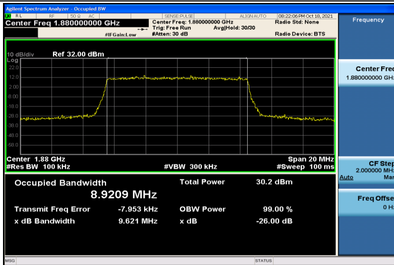
Band2-10MHz-QPSK-18900-50RB#0-8.9209
