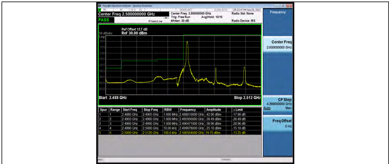
Band7-10MHz-QPSK-20800-50RB#0
