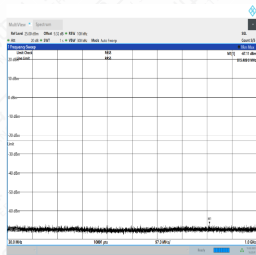
NTNV_N77-3450- 3550_PC2_30_20_H_TID2_NS_01_30_1000_#1
