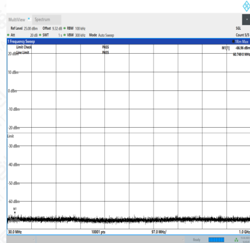
NTNV_N77-3450- 3550_PC2_30_60_L_TID4_NS_01_30_1000_#1
