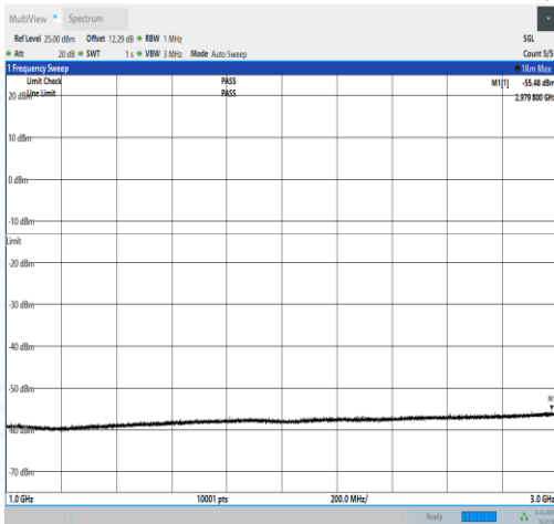
NTNV_N77-3450- 3550_PC2_30_20_L_TID4_NS_01_1000_3000_#1
