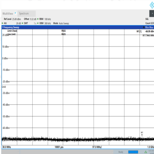
NTNV_N77-3450- 3550_PC2_30_60_L_TID1_NS_01_30_1000_#1
