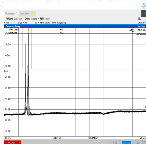
NTNV_N77-3450- 3550_PC2_30_60_L_TID4_NS_01_30_1000_#1
