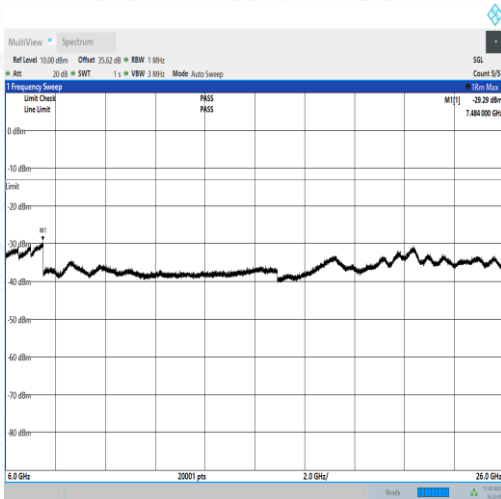
NTNV_N77-3450- 3550_PC2_30_20_L_TID4_NS_01_6000_26000_#1
