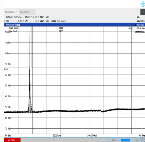
NTNV_N77-3450- 3550_PC2_30_20_H_TID2_NS_01_3000_6000_#1
