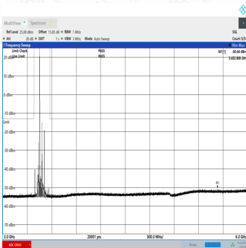
NTNV_N77-3450- 3550_PC2_30_60_L_TID1_NS_01_30_1000_#1
