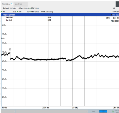
NTNV_N77-3450- 3550_PC2_30_20_M_TID4_NS_01_6000_26000_#1
