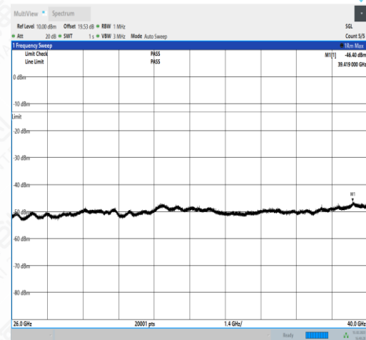
NTNV_N77-3450- 3550_PC2_30_60_L_TID2_NS_01_26000_40000_#1
