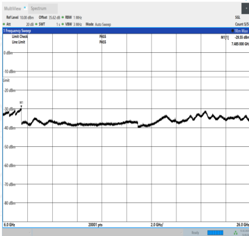
NTNV_N77-3450- 3550_PC2_30_60_M_TID2_NS_01_6000_26000_#1
