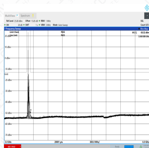
NTNV_N77-3450- 3550_PC2_30_20_M_TID2_NS_01_30_1000_#1
