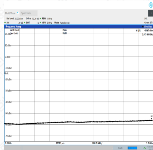
NTNV_N77-3450- 3550_PC2_30_60_L_TID1_NS_01_1000_3000_#1
