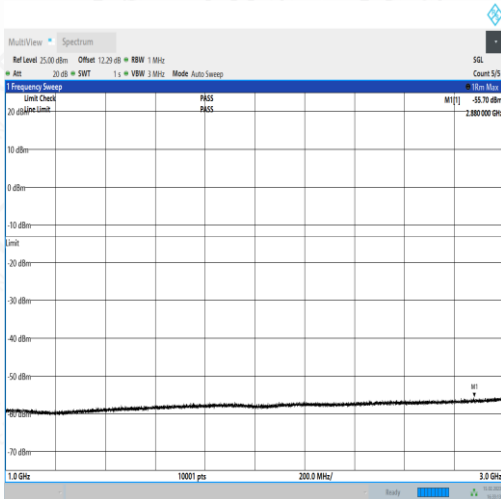
NTNV_N77-3450- 3550_PC2_30_20_H_TID2_NS_01_1000_3000_#1
