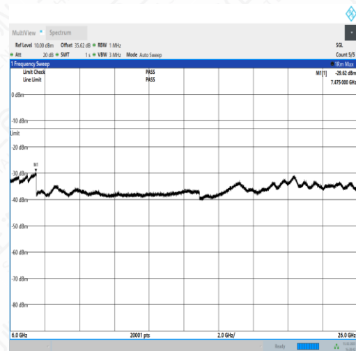
NTNV_N77-3450- 3550_PC2_30_60_L_TID1_NS_01_1000_3000_#1
