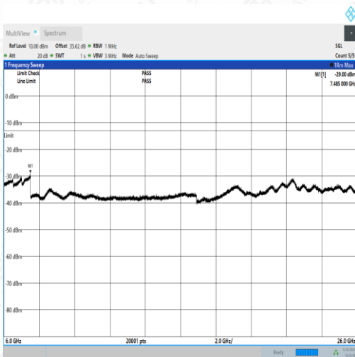
NTNV_N77-3450- 3550_PC2_30_20_H_TID2_NS_01_1000_3000_#1
