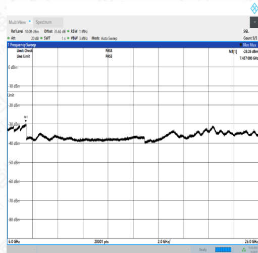
NTNV_N77-3450- 3550_PC2_30_20_M_TID3_NS_01_6000_26000_#1
